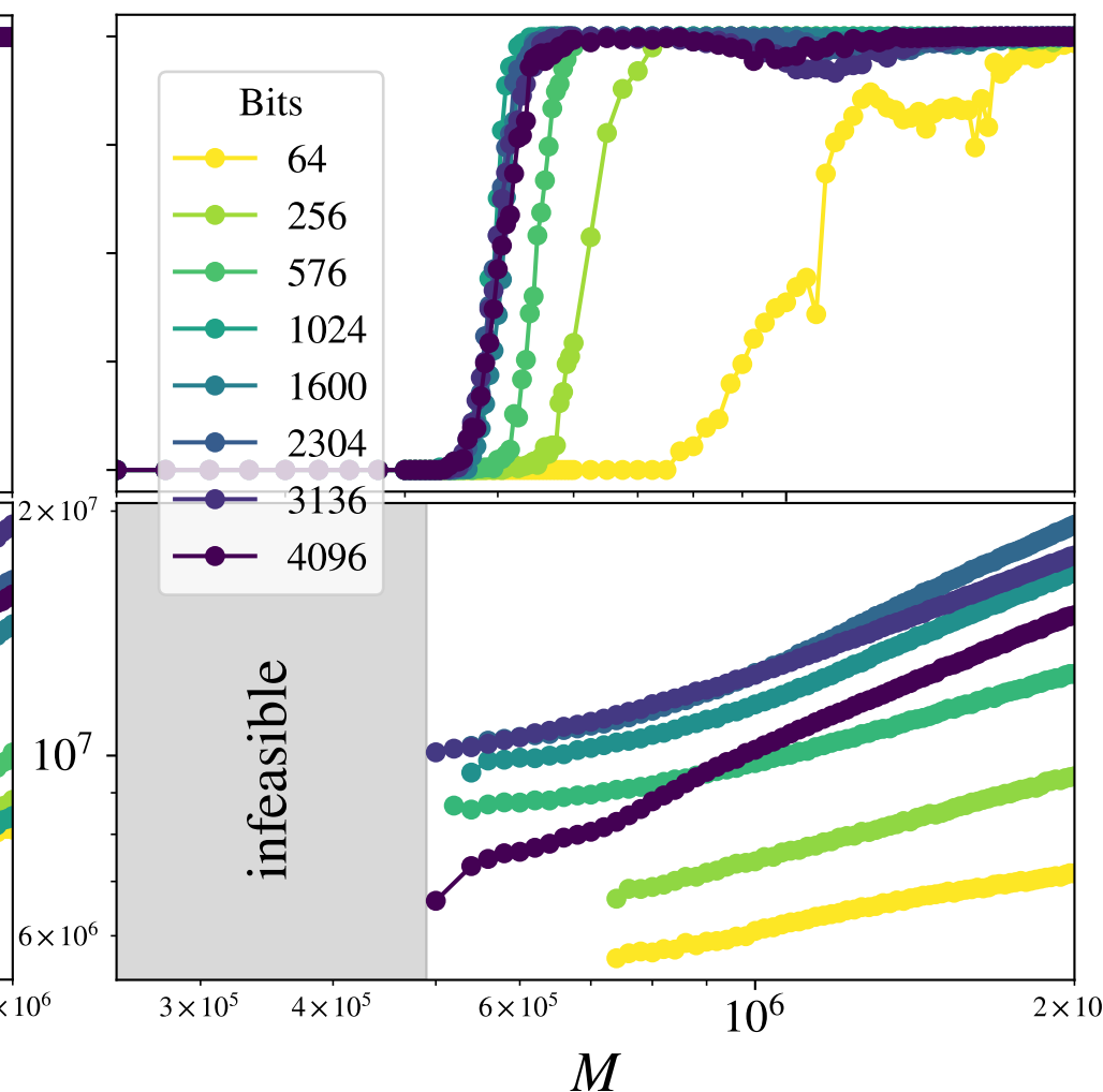
circle TSP
