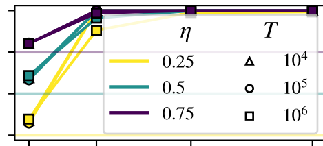
circle TSP
