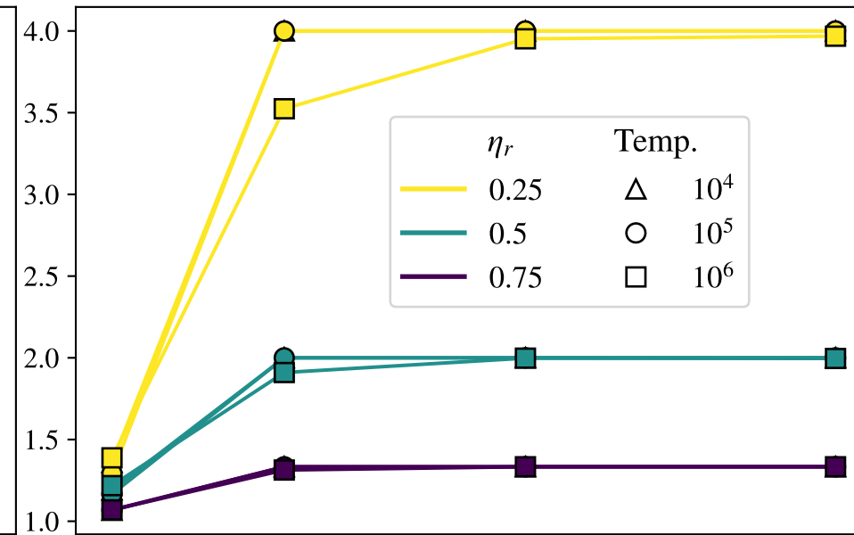
circle TSP
