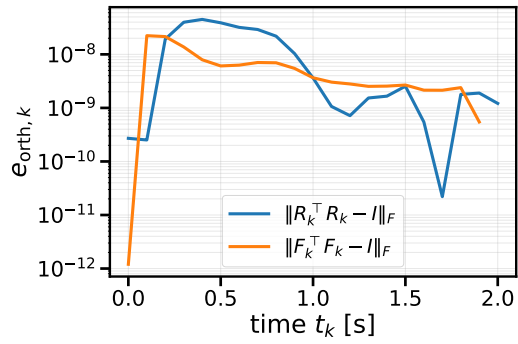
(d) Orthogonality errors e_{\text{orth},k}^P of \mathbf{R}_k, \mathbf{F}_k .
