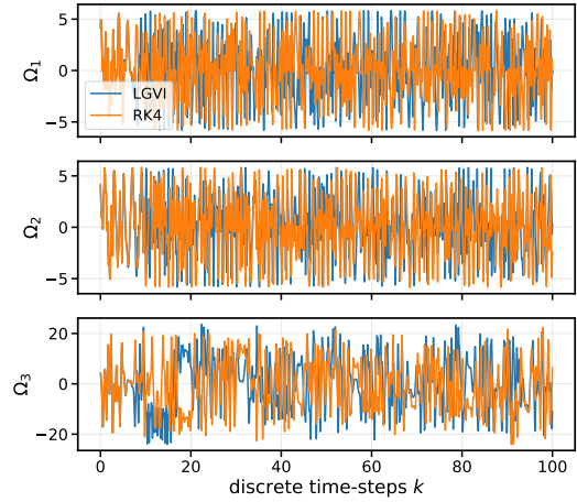
(d) Angular velocity components \boldsymbol{\Omega}_k .
