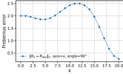
(c) Frobenius tracking error \|\mathbf{R}_k - \mathbf{R}_{\text{des}}\|_F .
