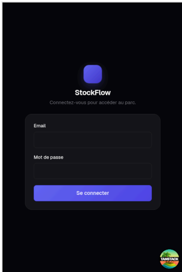
Connexion
