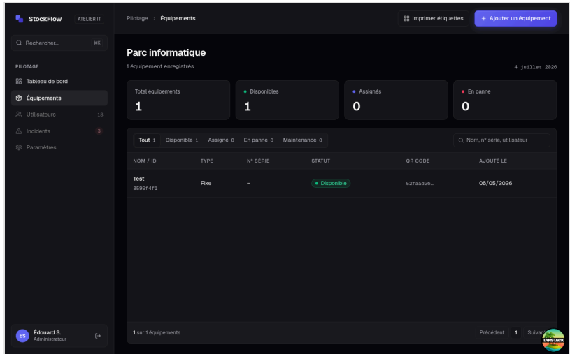
Inventaire (desktop)
