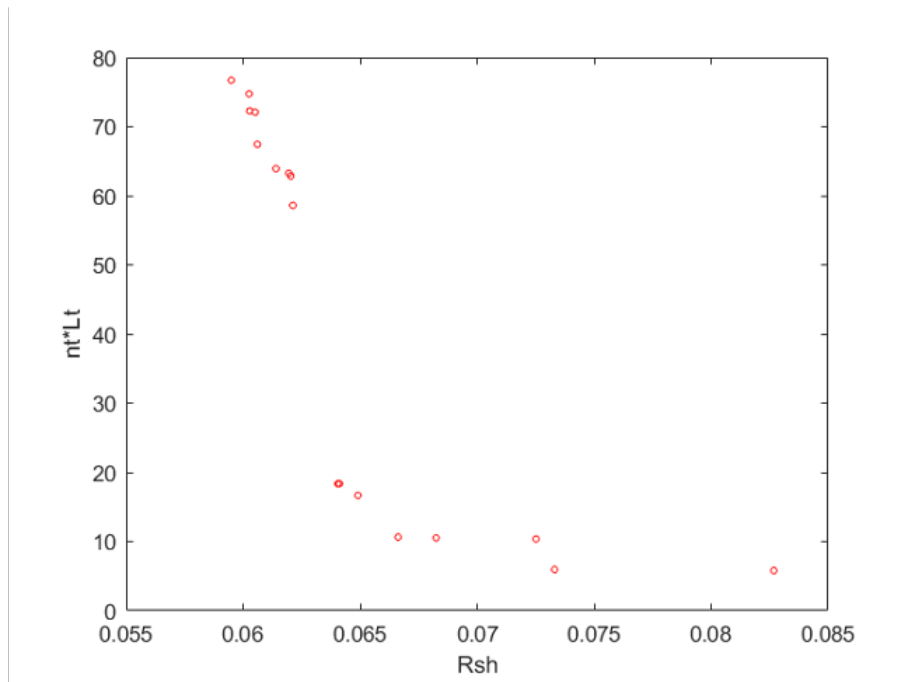
Figure 4.11: Front de Pareto entre R_{sh} et n_t \times L_t pour une surpuissance de 200%
