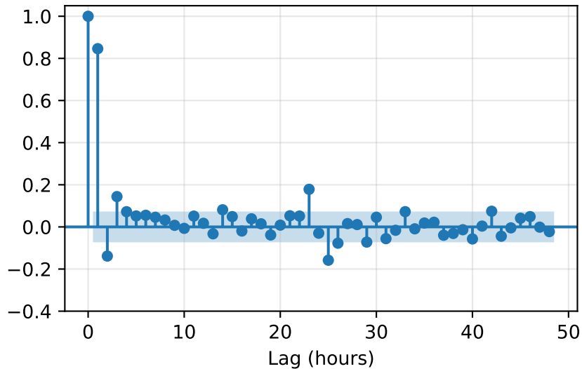
PACF
