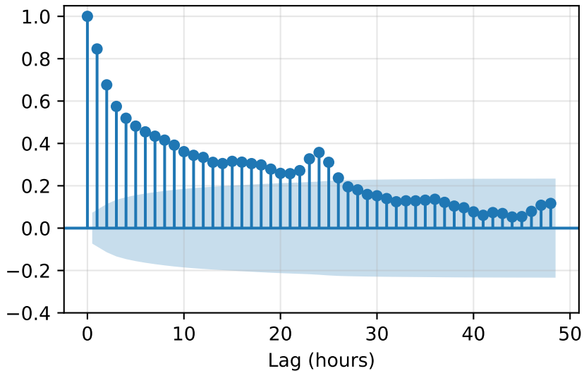
ACF
