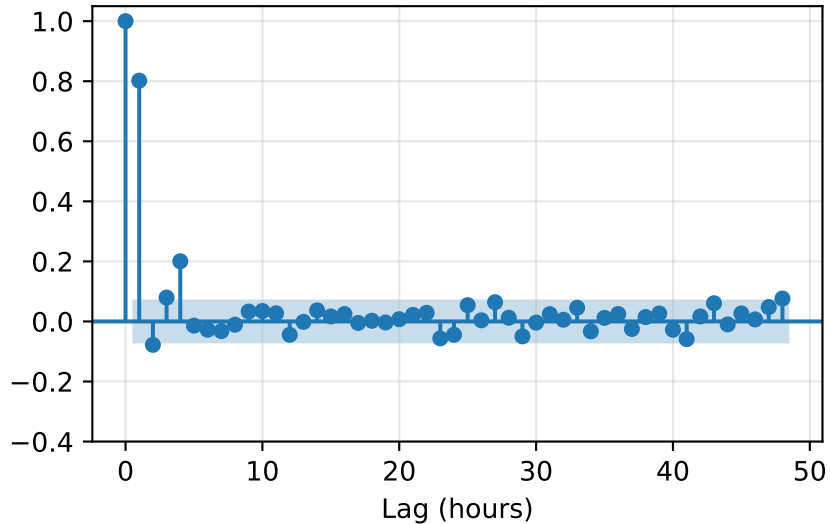
PACF
