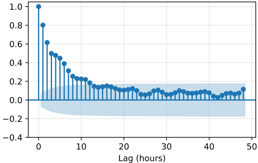
ACF
