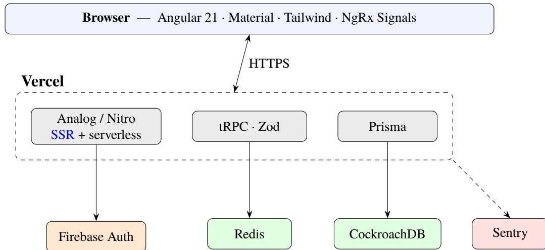
Figura 2: Arhitectura de ansamblu: browserul ( Angular ) comunică prin HTTPS cu platforma Vercel , care găzduiește runtime-ul Analog/Nitro ( SSR + funcții serverless), stratul tRPC (cu validare Zod ) și clientul Prisma . Persistența și serviciile transversale sunt gestionate extern: CockroachDB (date), Redis (cache, rate-limiting ), Firebase (autentificare) și Sentry (monitorizarea erorilor).
