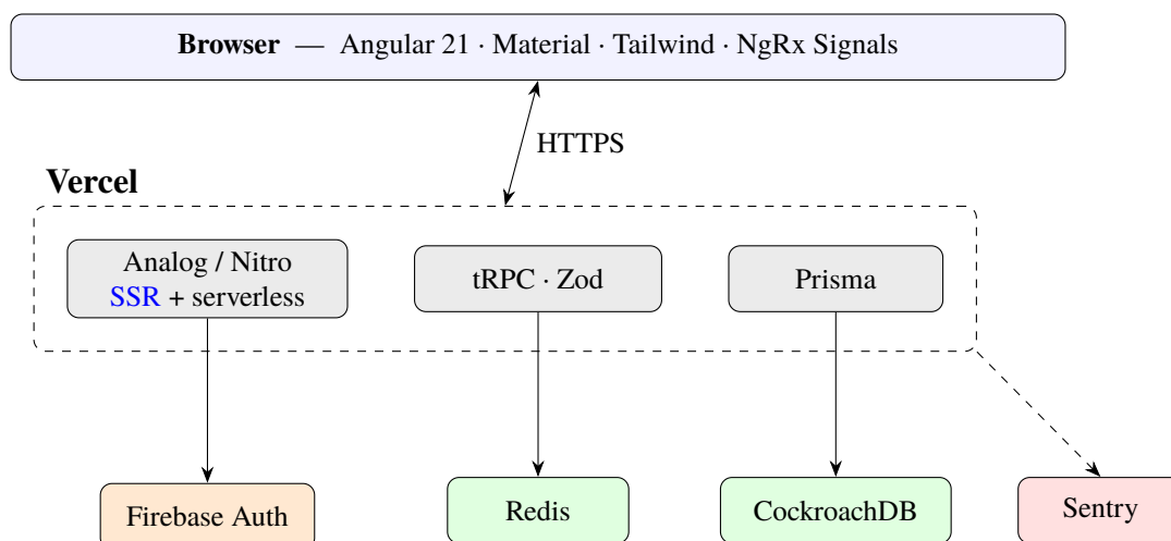
Figura 1: Arhitectura de ansamblu: browserul ( Angular ) comunică prin HTTPS cu platforma Vercel , care găzduiește runtime-ul Analog/Nitro ( SSR + funcții serverless), stratul tRPC (cu validare Zod ) și clientul Prisma . Persistența și serviciile transversale sunt gestionate extern: CockroachDB (date), Redis (cache, rate-limiting ), Firebase (autentificare) și Sentry (monitorizarea erorilor).
