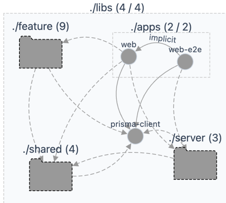
Figura 2: Graful de dependențe al proiectului (Nx), colapsat pe cele patru domenii de scope : feature (9 biblioteci), server (3), shared (4) și prisma-client , plus aplicațiile web și web-e2e . Săgețile redau relația de dependență; topologia este aciclică ( apps → feature → server , shared , prisma-client ), straturile inferioare neavând dependențe către cele superioare.
