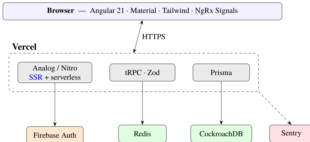
Figura 1: Arhitectura de ansamblu: browserul ( Angular ) comunică prin HTTPS cu platforma Vercel , care găzduiește runtime-ul Analog/Nitro ( SSR + funcții serverless), stratul tRPC (cu validare Zod ) și clientul Prisma . Persistența și serviciile transversale sunt gestionate extern: CockroachDB (date), Redis (cache, rate-limiting ), Firebase (autentificare) și Sentry (monitorizarea erorilor).
