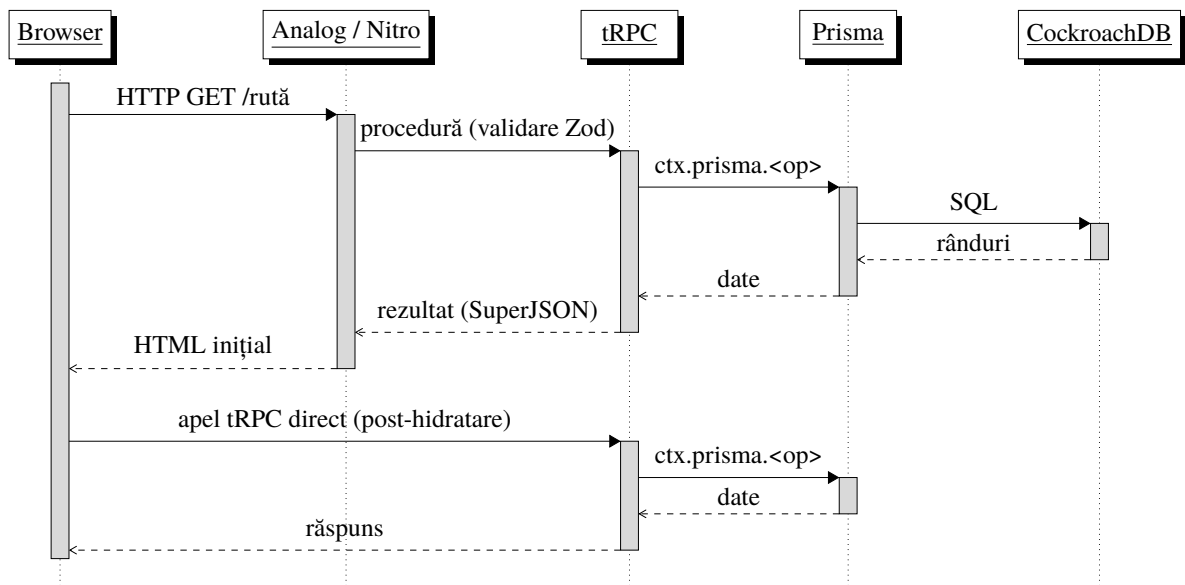
Figura 3: Diagrama de secvență a unei cereri. Randare inițială (SSR): cererea HTTP ajunge la runtime-ul Analog/Nitro , care interoghează persistența prin straturile tRPC (cu validare Zod ) → Prisma → CockroachDB și returnează HTML-ul inițial. Interacțiune ulterioară: după hidratare, apelurile pleacă direct din browser către tRPC , fără o nouă randare pe server.
