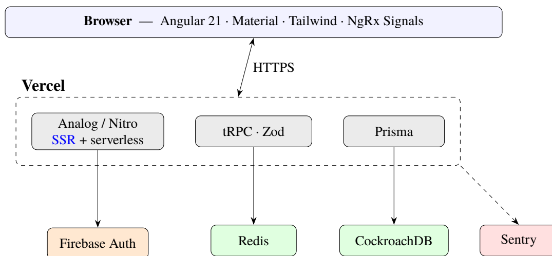
Figura 1: Arhitectura de ansamblu: browserul ( Angular ) comunică prin HTTPS cu platforma Vercel , care găzduiește runtime-ul Analog/Nitro (SSR + funcții serverless), stratul tRPC (cu validare Zod ) și clientul Prisma . Persistența și serviciile transversale sunt gestionate extern: CockroachDB (date), Redis (cache, rate-limiting ), Firebase (autentificare) și Sentry (monitorizarea erorilor).
