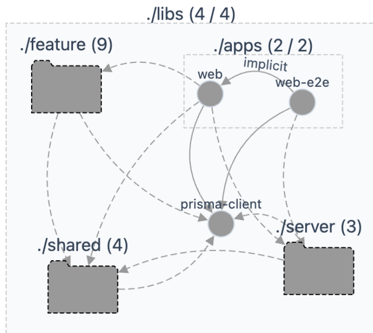
Figura 1: Graful de dependențe al proiectului (Nx), colapsat pe cele patru domenii de scope : feature (9 biblioteci), server (3), shared (4) și prisma-client, plus aplicațiile web și web-e2e. Săgețile redau relația de dependență; topologia este aciclică (apps → feature → server, shared, prisma-client), straturile inferioare neavând dependențe către cele superioare.
