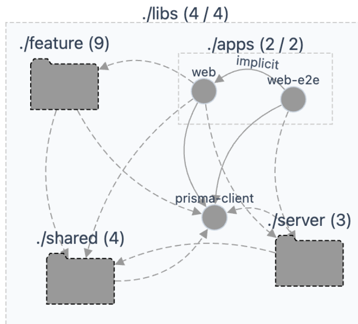
Figura 3: Graful de dependențe al proiectului ( Nx ), colapsat pe cele patru domenii de scope : feature (9 biblioteci), server (3), shared (4) și prisma-client , plus aplicațiile web și web-e2e . Săgețile redau relația de dependență; topologia este aciclică ( apps → feature → server , shared , prisma-client ), straturile inferioare neavând dependențe către cele superioare.
