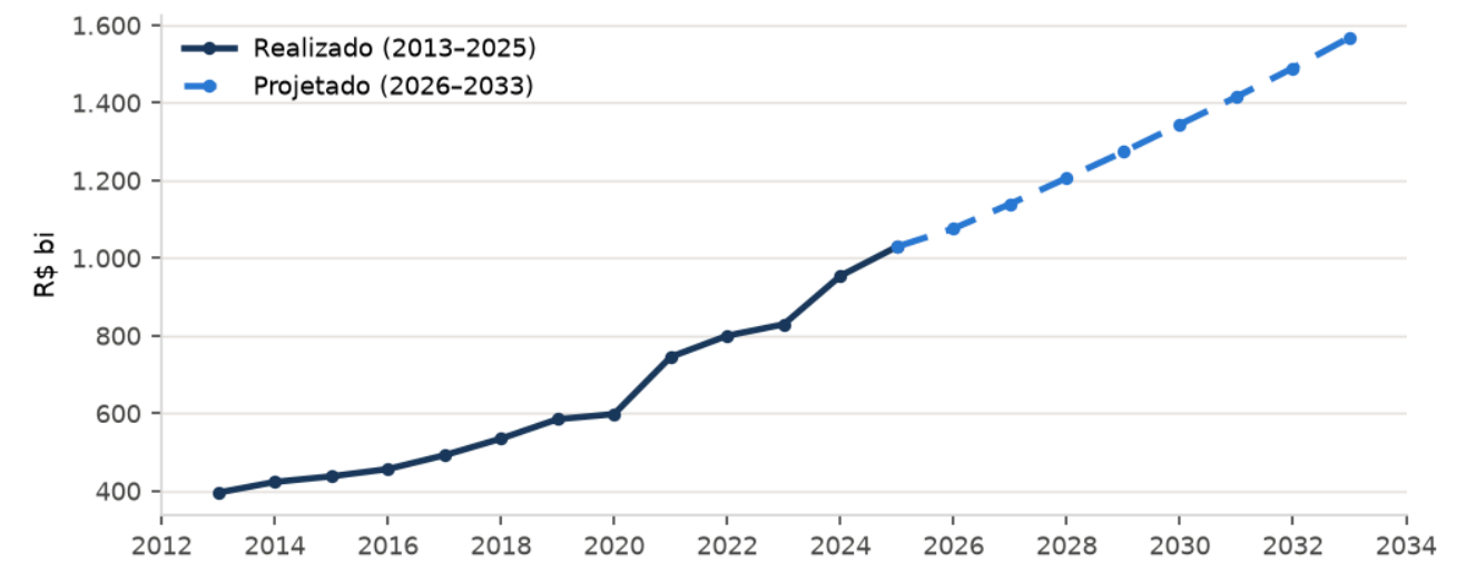
Arrecadação total de ICMS+ISS, Brasil (R$ bi, nominal). A linha tracejada, a partir de 2026, é a projeção descrita na Seção 4.
