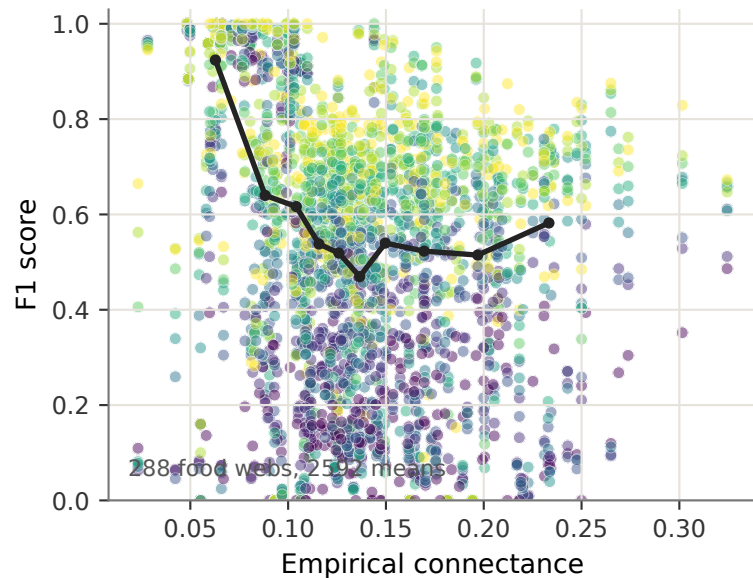
F1 score
