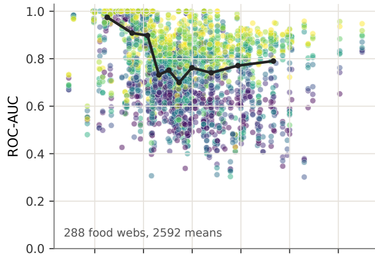
ROC-AUC
