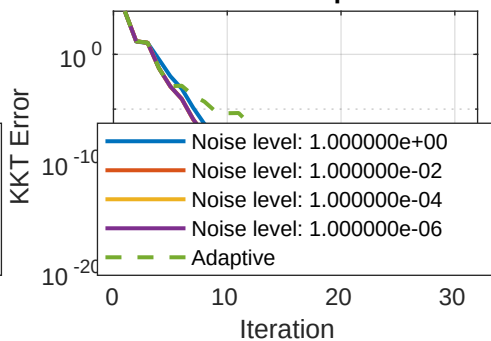
Matrix: exp
