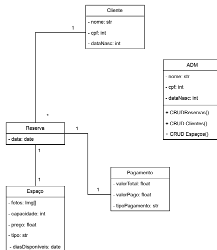
Figura 2: Diagrama de Classes do Sistema
