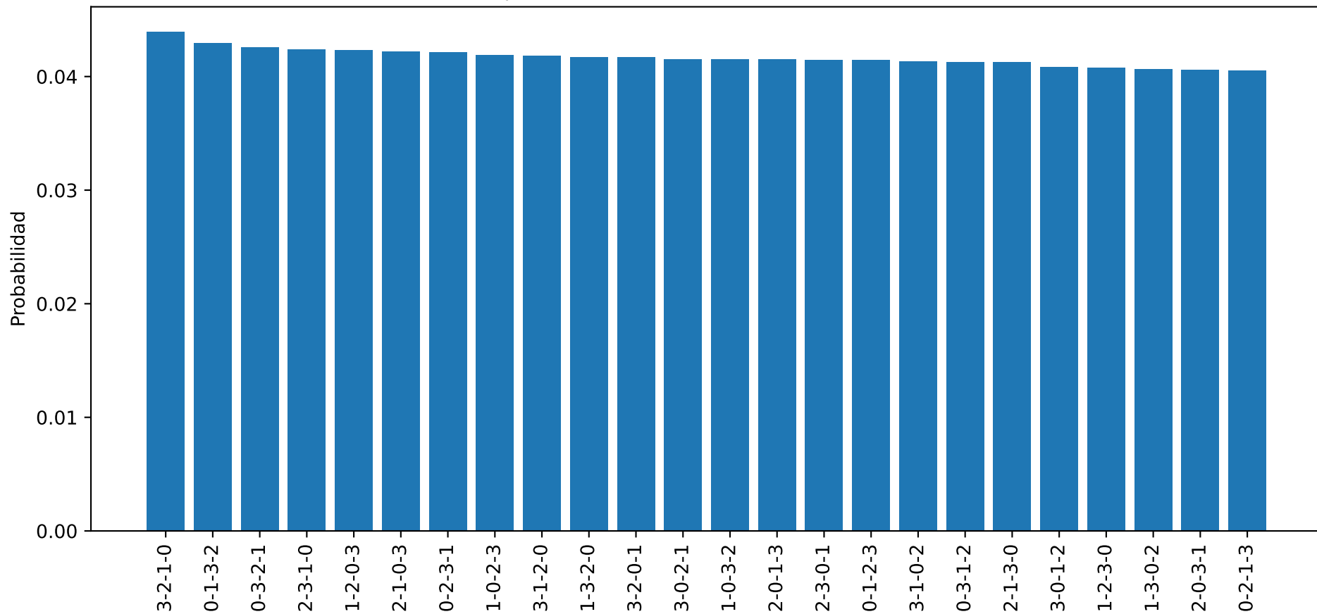
Distribución de patrones ordinales ( m=4 , \tau=1 ) — ventanas=49997
