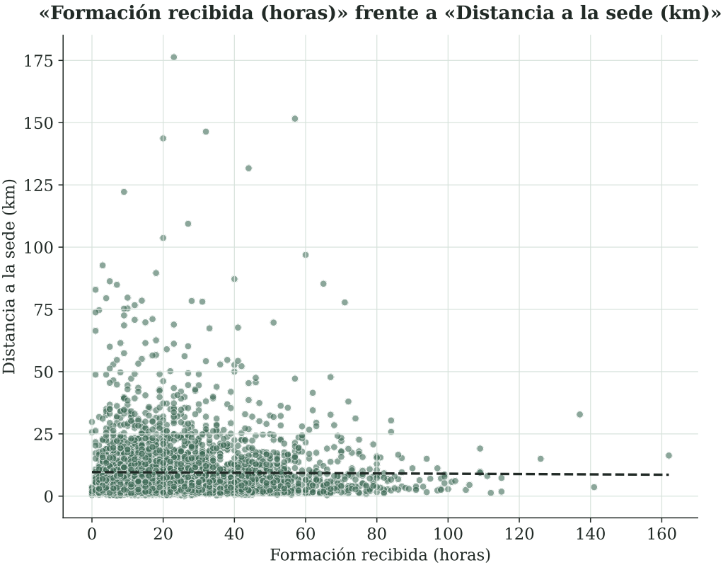
Figura 8. «Formación recibida (horas)» frente a «Distancia a la sede (km)».
