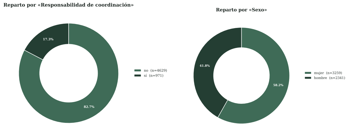
Figura 6. Reparto de registros por «Responsabilidad de coordinación» (izquierda) y por «Sexo» (derecha).
