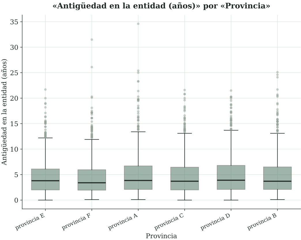
Figura 9. «Antigüedad en la entidad (años)» desagregado por «Provincia».
