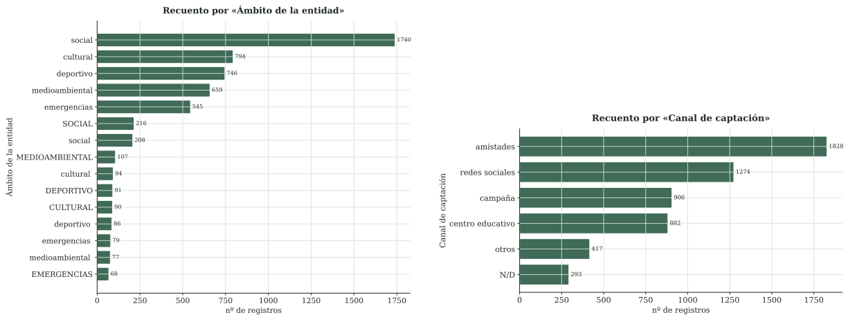
Figura 5. Recuento de registros por «Ámbito de la entidad» (izquierda) y por «Canal de captación» (derecha).
