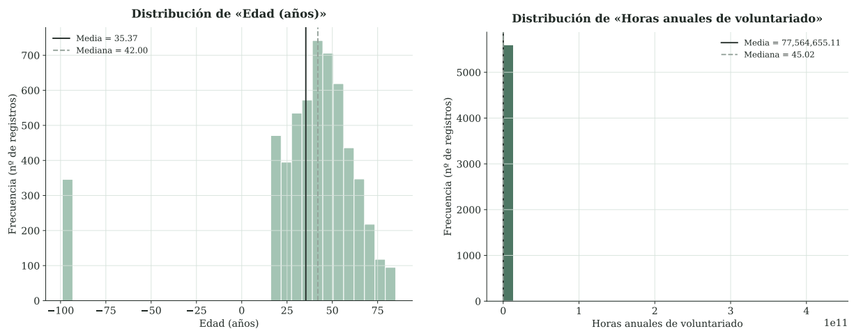
Figura 3. Distribución de «Edad (años)» (izquierda) y de «Horas anuales de voluntariado» (derecha).
