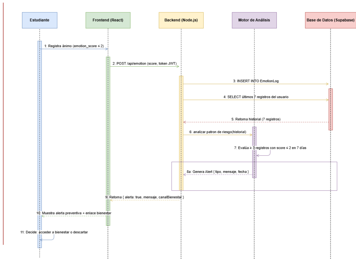
Figura 7. Diagrama de Secuencia — Generación de Alertas de Riesgo
