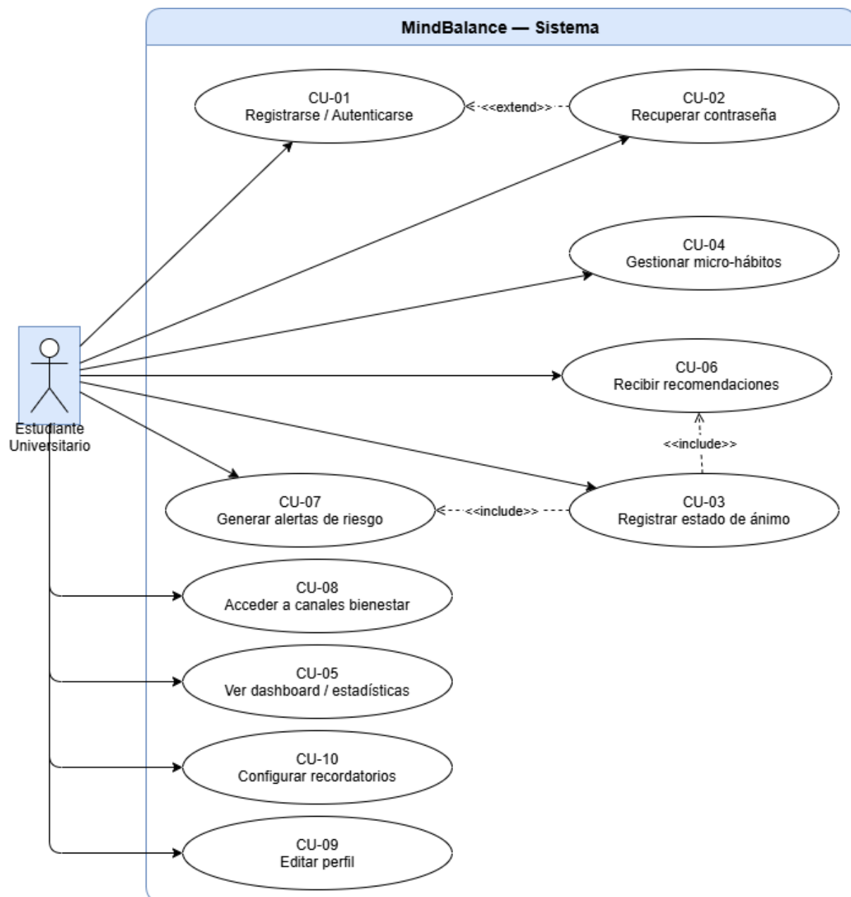
Figura 3. Diagrama de Casos de Uso — MindBalance
