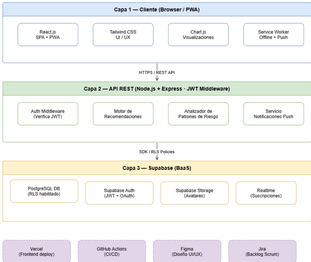
Figura 4. Diagrama de Arquitectura del Sistema — MindBalance
