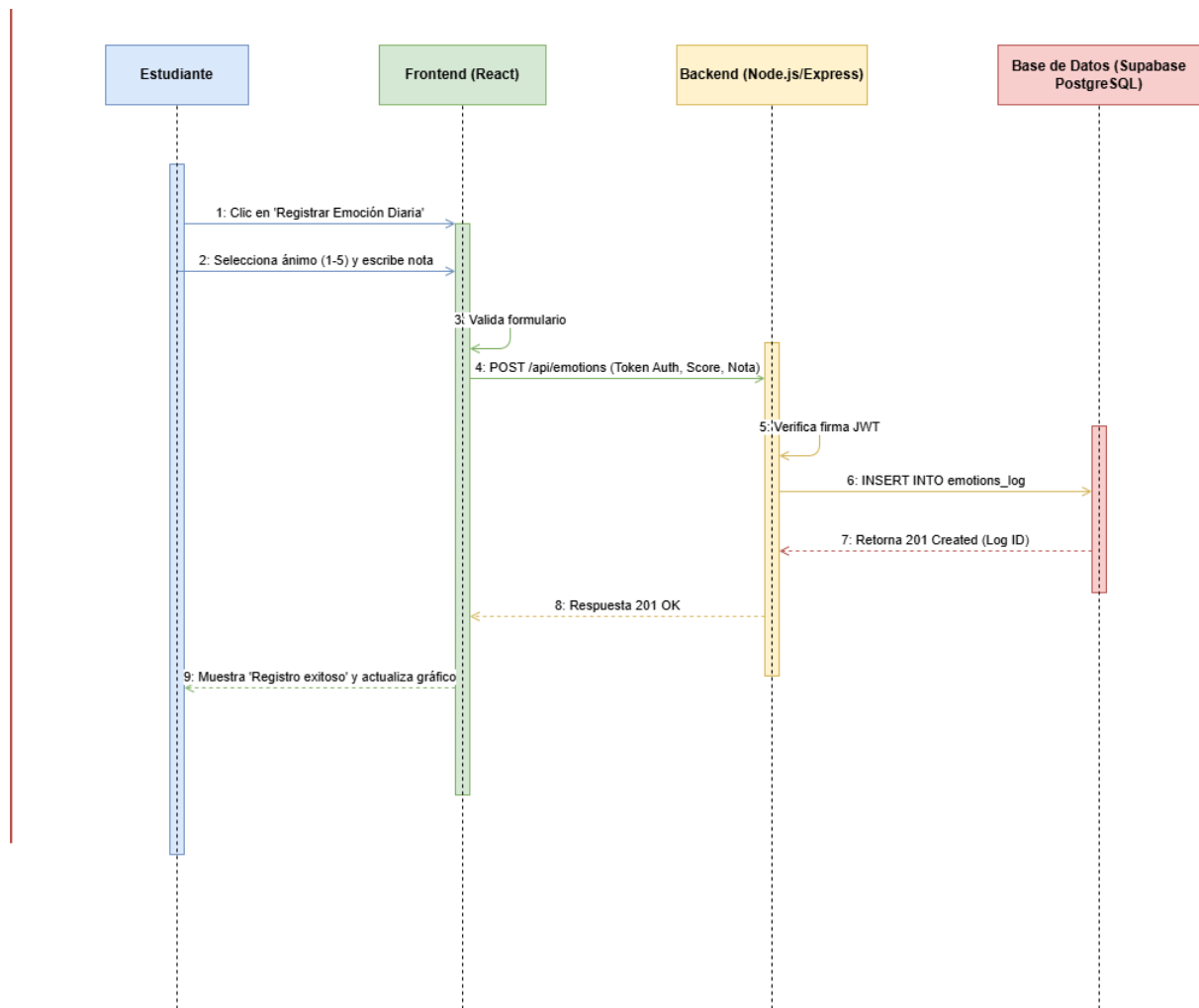
Figura 6. Diagrama de Secuencia — Flujo de Registro Emocional
