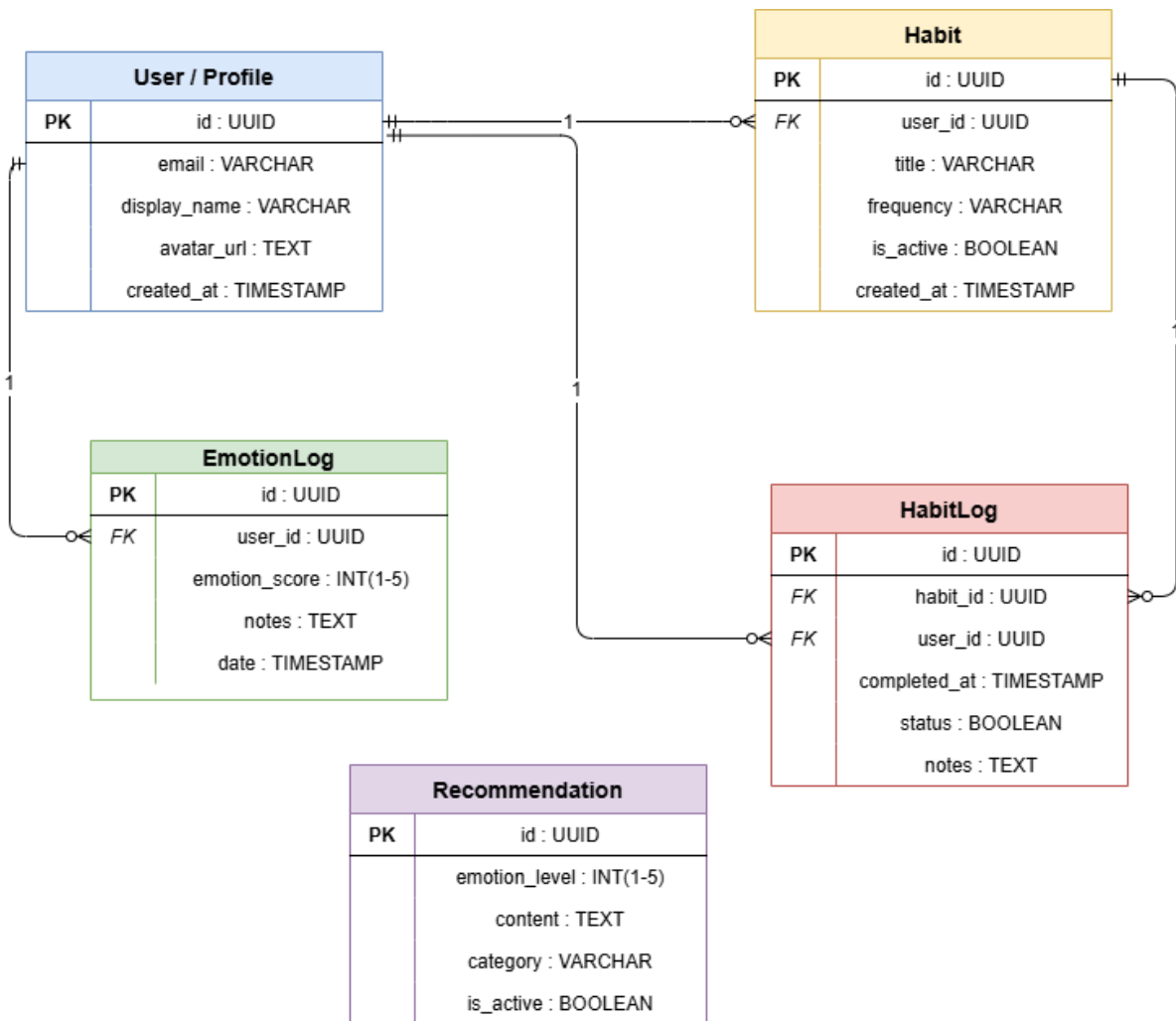
Figura 5. Diagrama Entidad-Relación (Modelo Lógico PostgreSQL)
