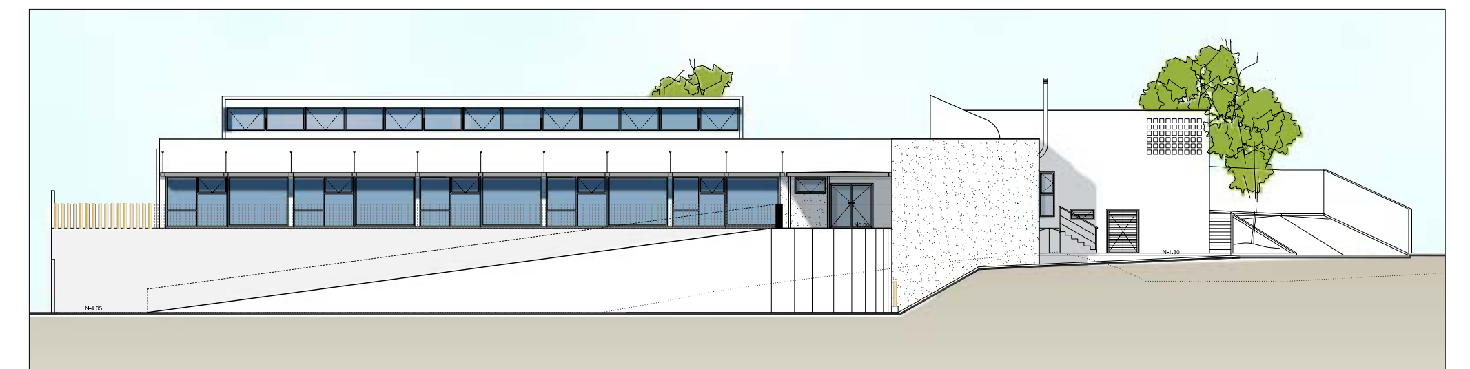
ALÇAT EST E 1:250
