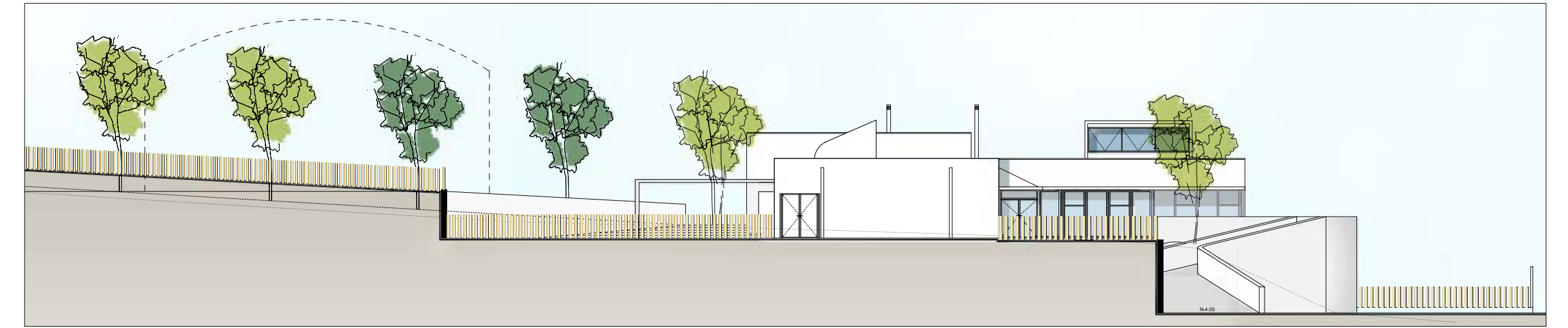
ALÇAT SUD E 1:250
