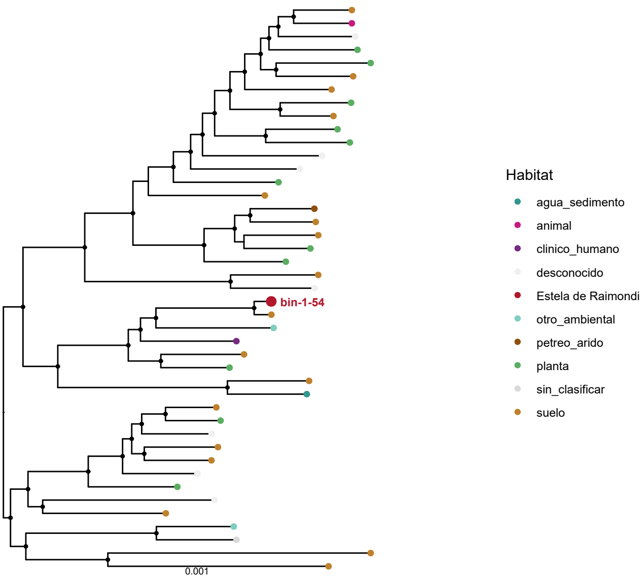
Maxima verosimilitud (IQ-TREE 3) sobre el core; punto negro: UFBoot >= 95.
