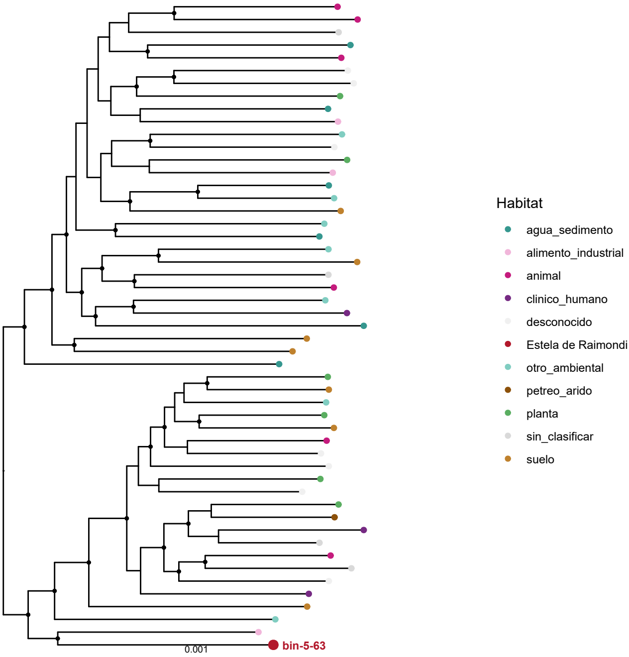
Maxima verosimilitud (IQ-TREE 3) sobre el core; punto negro: UFBoot >= 95.
