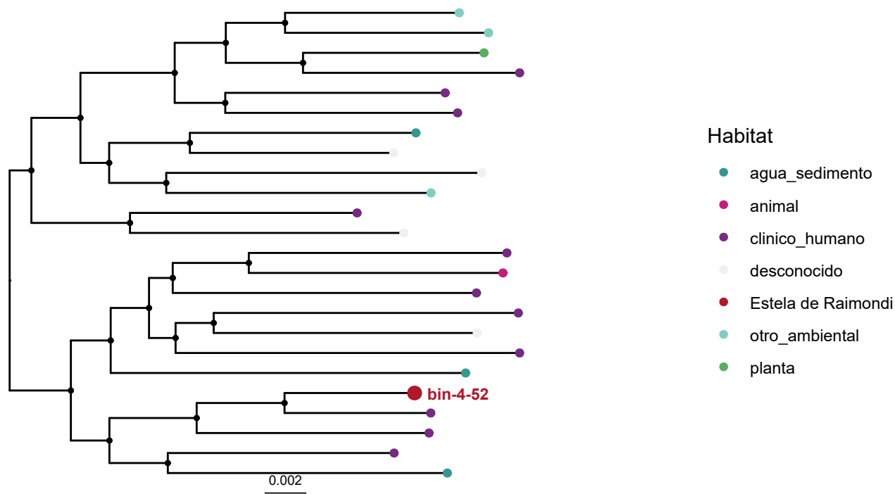
Maxima verosimilitud (IQ-TREE 3) sobre el core; punto negro: UFBoot >= 95.
