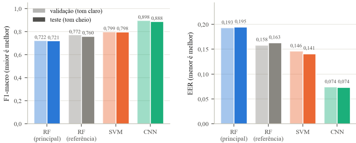
Figura 10 – F1-macro e EER dos quatro modelos na validação e no teste, com o limiar selecionado na validação
