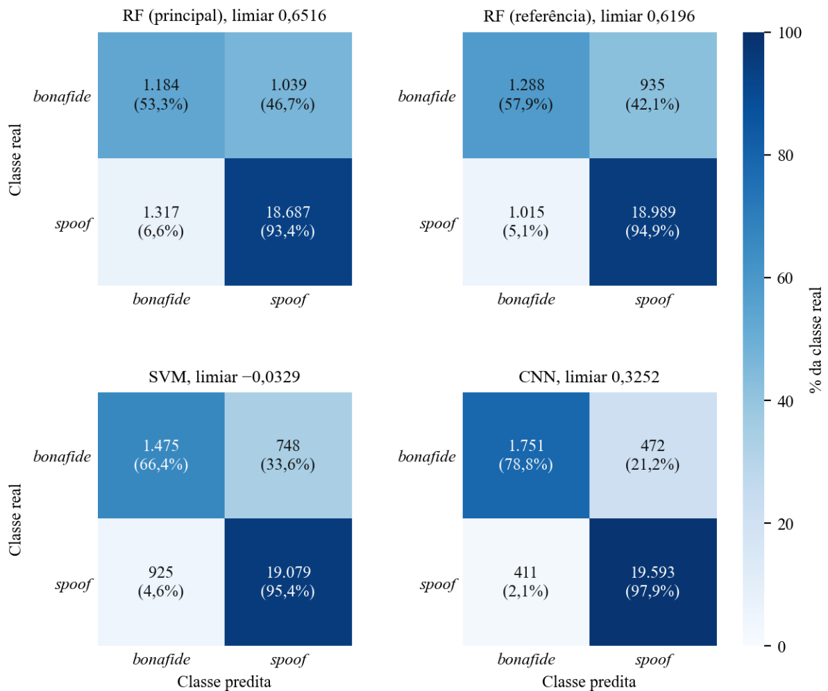
Figura 9 – Matrizes de confusão dos quatro modelos no teste (n = 22.227), com o limiar selecionado na validação: contagem e percentual da classe real em cada célula
