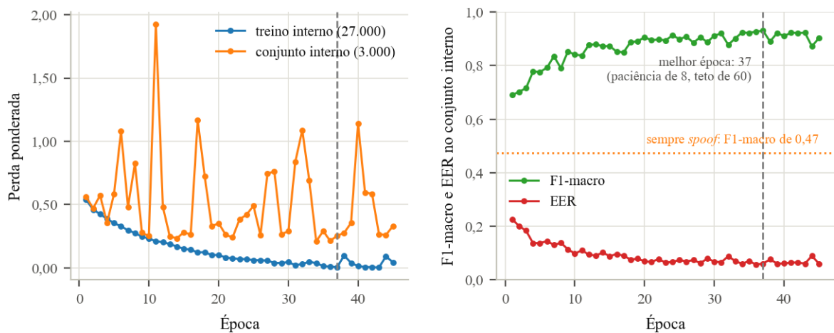
Figura 7 – Curvas de treino da configuração escolhida da CNN: perda ponderada no treino interno (27.000) e no conjunto interno (3.000), à esquerda, e F1-macro e EER no conjunto interno, à direita
