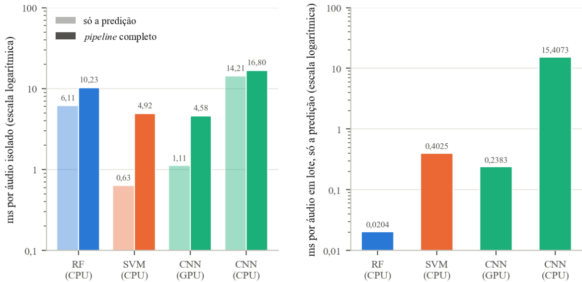
Figura 13 – Custo de inferência nos quatro arranjos: por áudio isolado (só a predição e pipeline completo) e em lote (só a predição), em escala logarítmica
