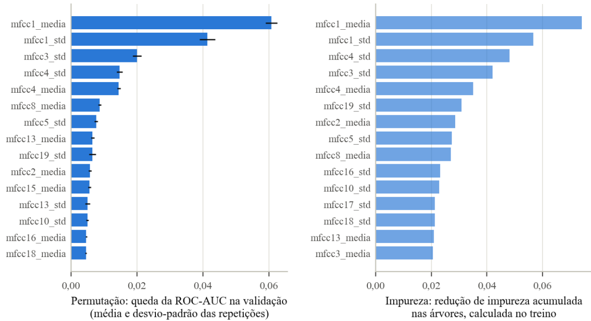
Figura 14 – Importância das características no RF principal: por permutação na validação e por redução de impureza
