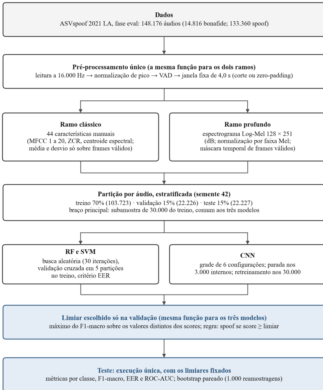
Figura 1 – Fluxograma do protocolo experimental
