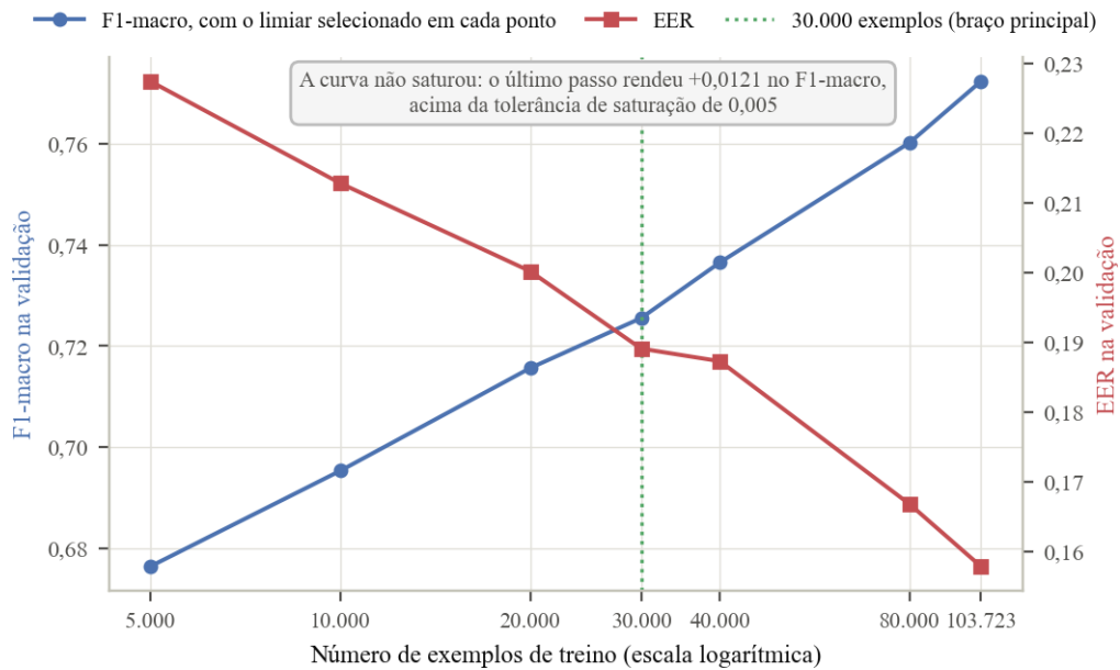
Figura 4 – Curva de aprendizado do RF ajustado na validação, com as características congeladas e o limiar selecionado em cada ponto
