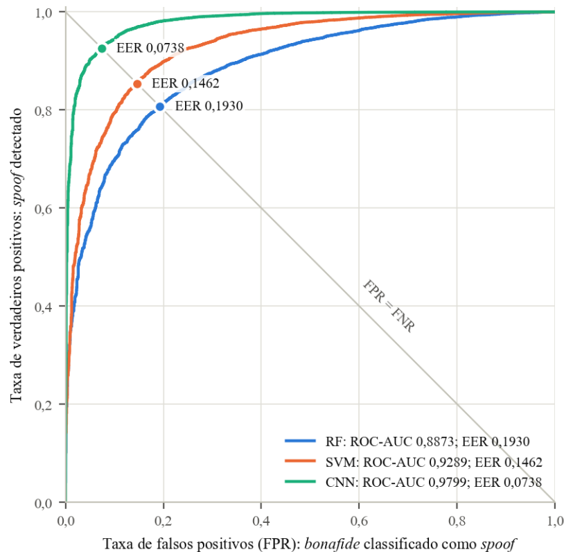
Figura 8 – Curvas ROC dos três modelos do braço principal na validação ( n = 22.226 ), com o EER marcado no cruzamento com a reta FPR = FNR
