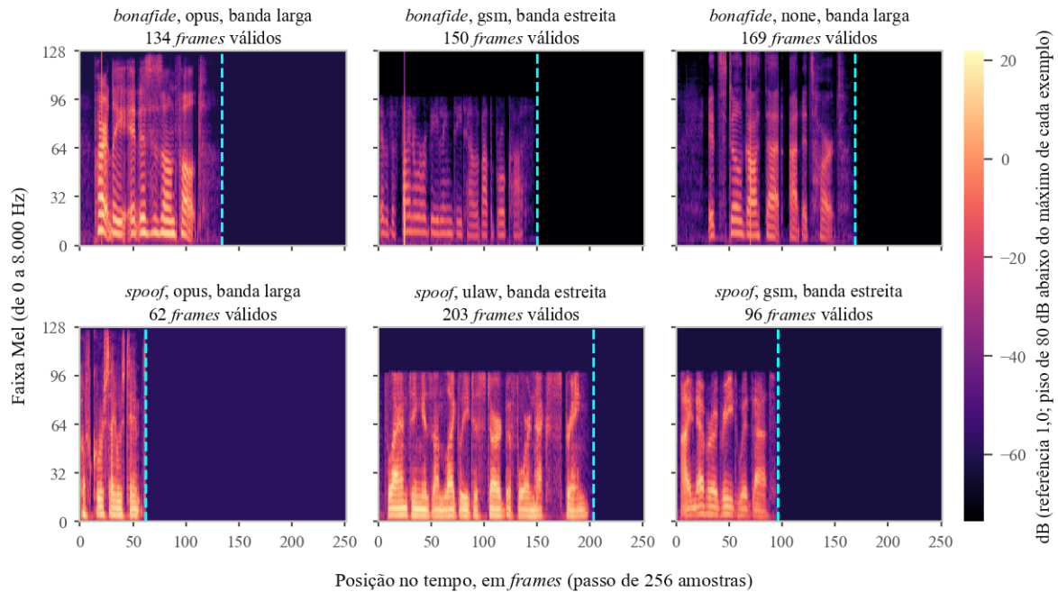
Figura 5 – Espectrogramas Log-Mel crus do piloto do gerador, com três exemplos bonafide (acima) e três spoof (abaixo), de banda larga e estreita; a linha tracejada marca o fim dos frames válidos
