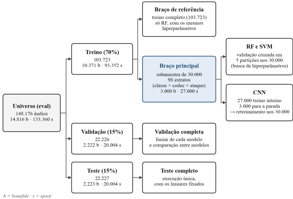
Figura 2 – Partição dos dados, braços do experimento e ponto em que cada modelo usa o treino
