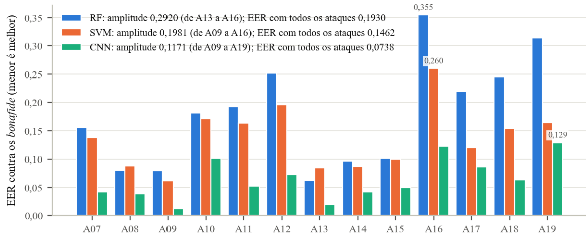
Figura 11 – EER por sistema de ataque (A07 a A19) dos três modelos do braço principal na validação (n = 22.226)
