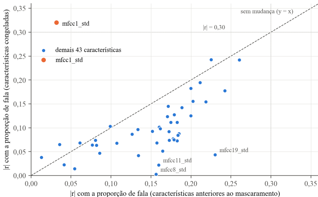
Figura 3 – Correlação absoluta de cada característica com a proporção de fala, antes e depois do mascaramento do padding (fase eval )
