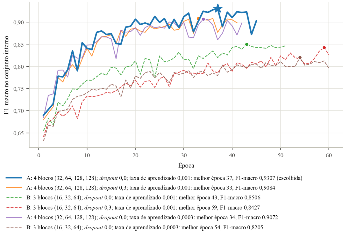
Figura 6 – F1-macro no conjunto interno de parada antecipada, por época, nas seis configurações da grade da CNN (a estrela marca a melhor época da configuração escolhida)
