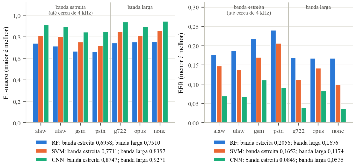
Figura 12 – F1-macro e EER por codec dos três modelos do braço principal na validação (n = 22.226), com o limiar do protocolo
