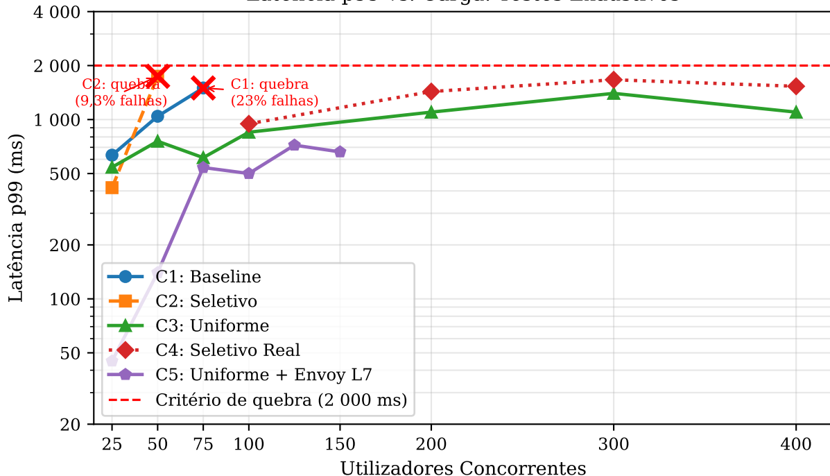
Latência p99 vs. Carga: Testes Exaustivos
