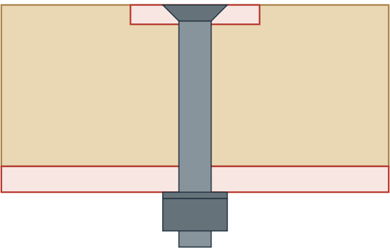
Šķērsgriezums 1:1,67
