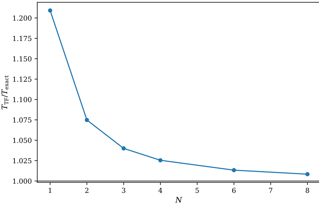
Thomas-Fermi kinetic energy
