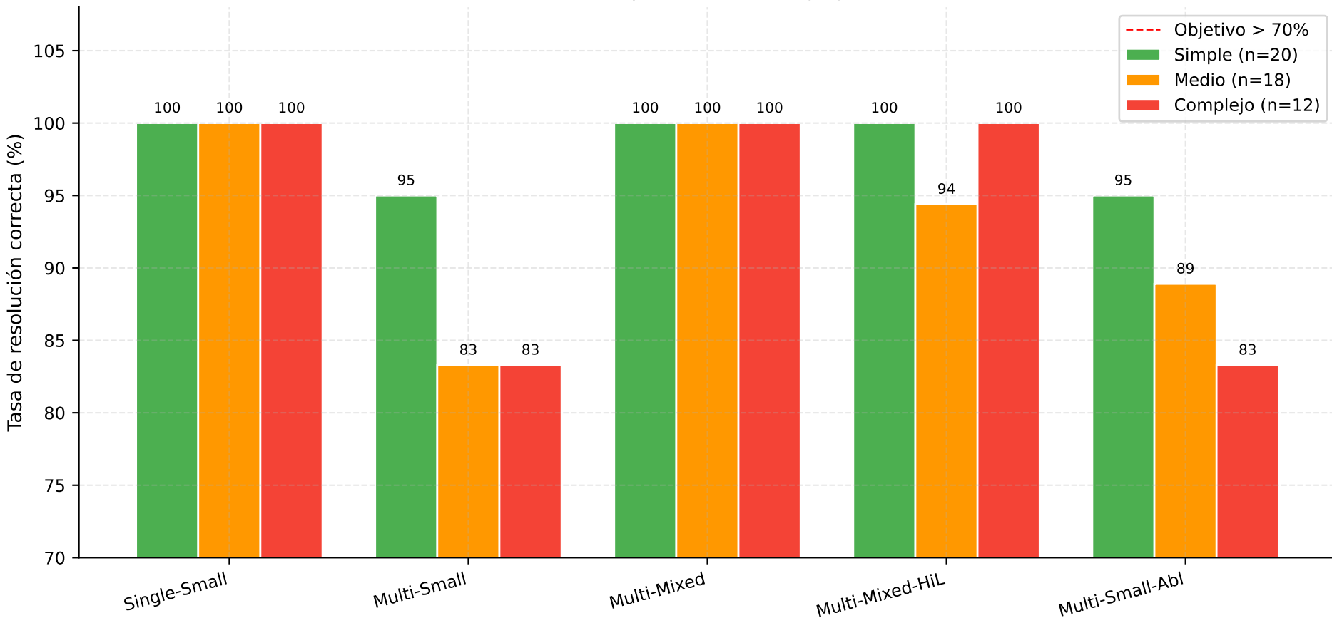
Tasa de resolución por nivel de complejidad del caso
