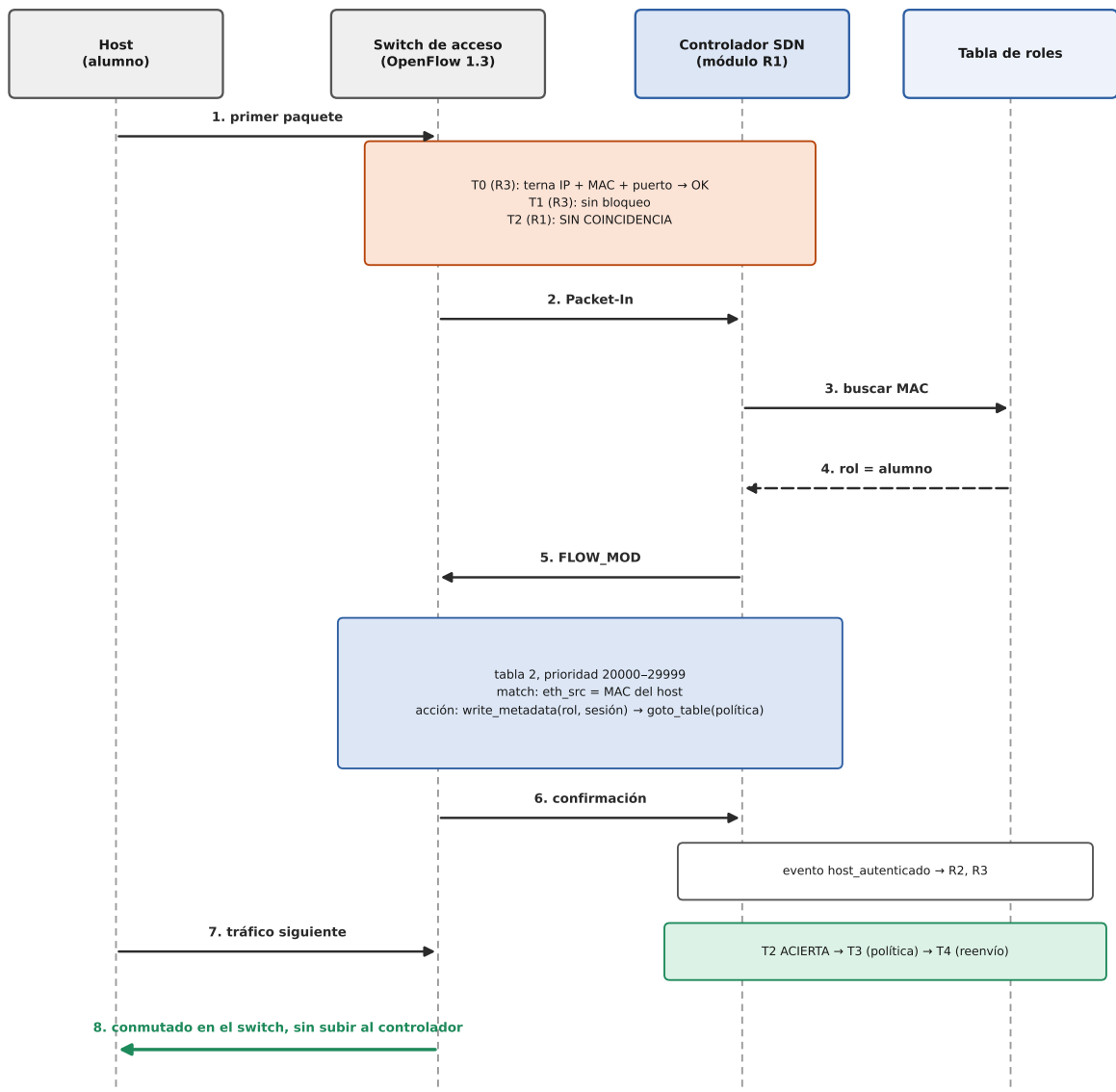
Figura 2: Secuencia de autenticación: desde el primer paquete hasta la instalación de la regla de rol.
