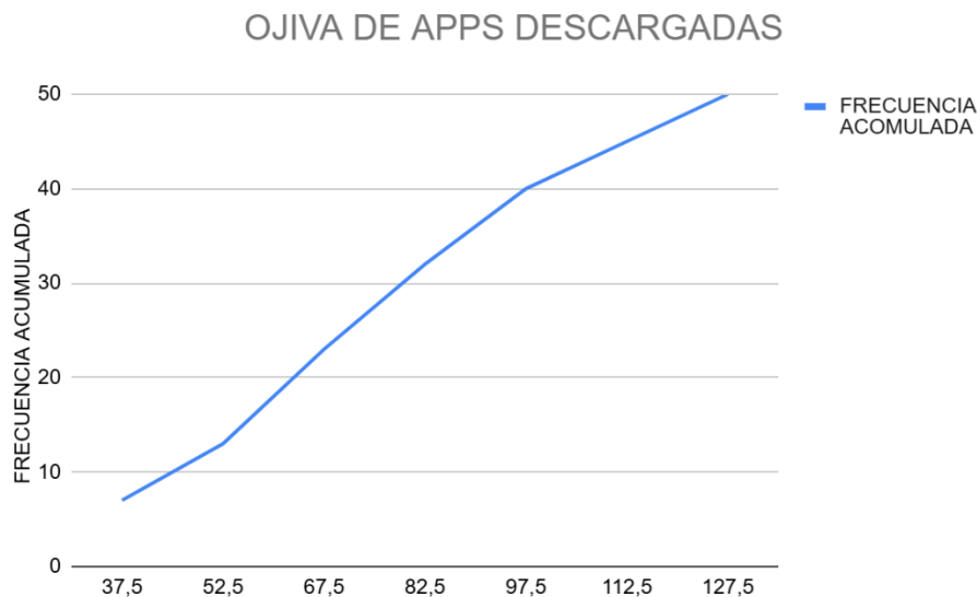
Figura 4: Ojiva de Apps Descargadas.
