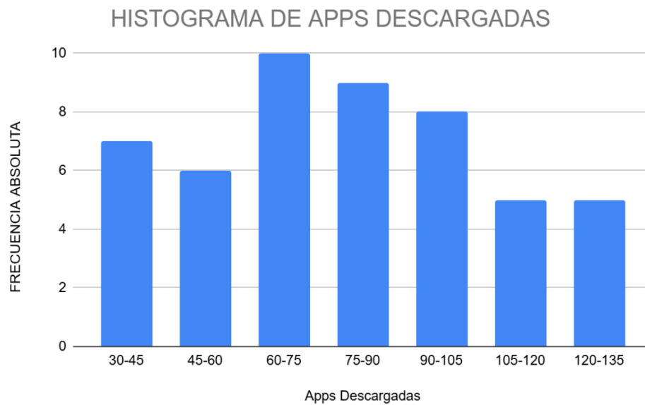
Figura 2: Histograma de frecuencia para Apps Descargadas.
