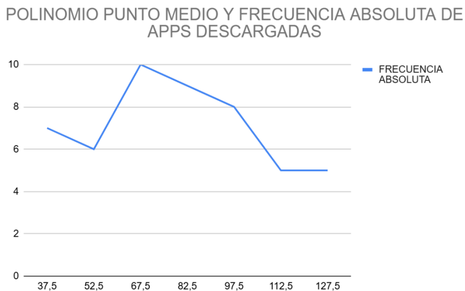
Figura 3: Polinomio de frecuencia de Apps Descargadas.
