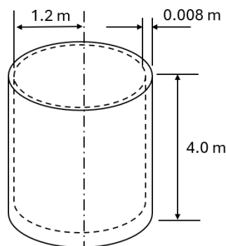
Figura: Tanque cilíndrico vertical com tampas planas
