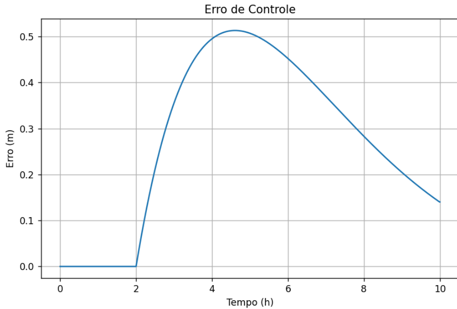
Figura 2: Resposta temporal do erro de controle, definido por e(t) = h(t) - h_{SP} . O aumento da vazão de alimentação provoca um desvio da interface água-óleo em relação ao valor desejado. O controlador PI atua continuamente sobre a válvula de saída de água para reduzir esse erro, fazendo com que o sistema retorne ao ponto de operação especificado.
