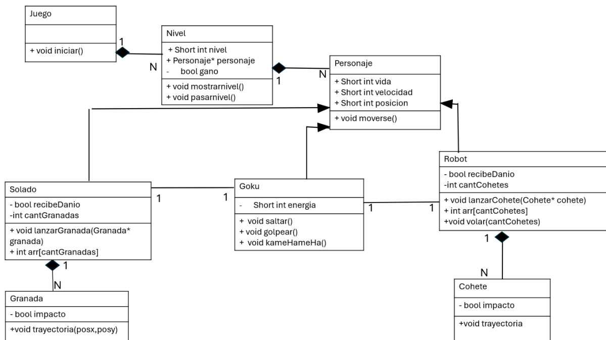
Figura 1: Diagrama de clases UML original para el videojuego.
