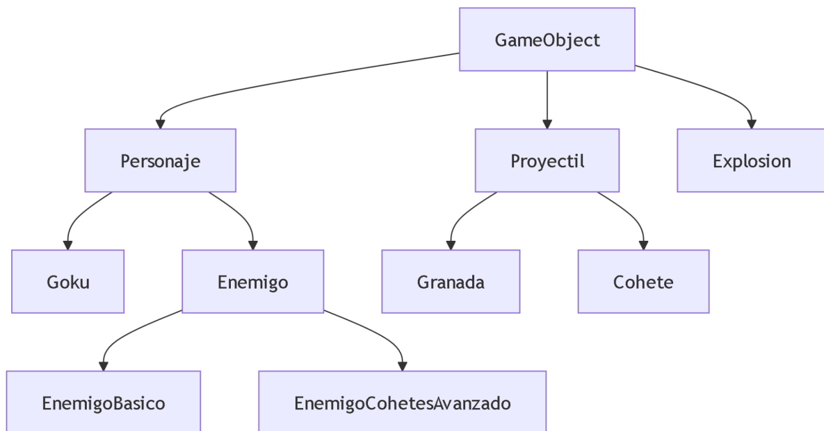
Figura 2: Diagrama de clases Básico para el videojuego.
