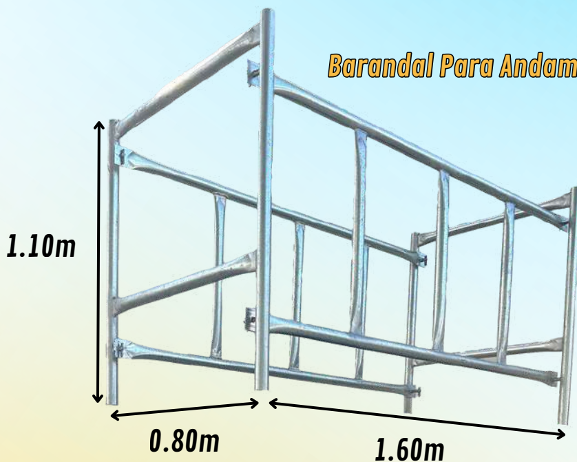
Barandal Para Andamio SPL-5
