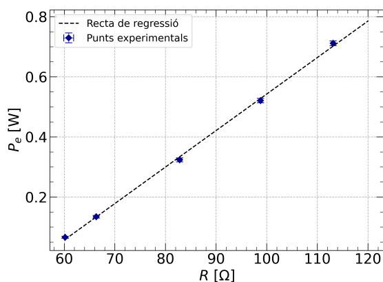
Figura 3: Representació i regressió lineal ( y = ax + b ) dels primers cinc punts experimentals de la gràfica P_e vs R . Coeficients de regressió: a = (12, 14 \pm 0, 22) \cdot 10^{-3} \text{ W}/\Omega , b = (-0, 672 \pm 0, 019) \text{ W} . Regressió amb un coeficient de r^2 = 0, 999 .
