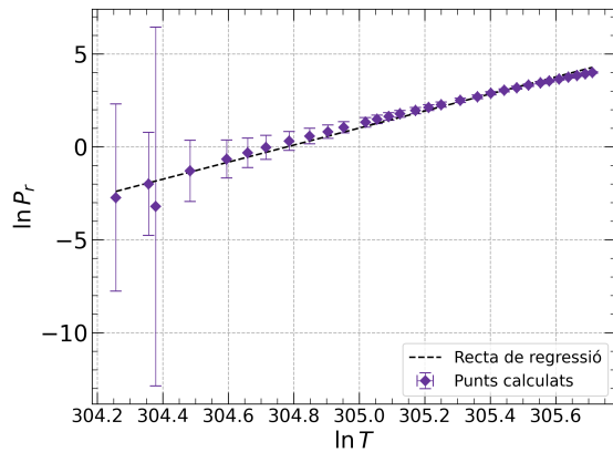
Figura 8: Representació i regressió lineal ( y = ax + b ) de \ln P_r vs \ln T per a les dades de la segona regió sense treure outliers. Coeficients de regressió: a = 4,59 \pm 0,13 , b = -1397 \pm 40 .
