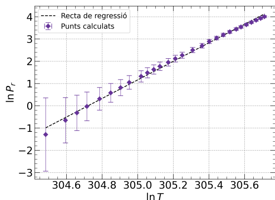
Figura 5: Representació i regressió lineal ( y = ax + b ) de \ln P_r vs \ln T per a les dades de la segona regió. No s'han tingut en compte els primers 4 punts pertanyents a la regió (veure Annex). Coeficients de regressió: a = 4,169 \pm 0,049 , b = -1270 \pm 15 . Regressió amb un coeficient de r^2 = 0,996
