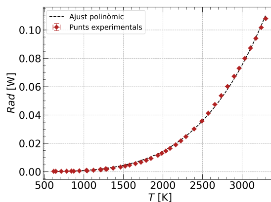
Figura 6: Representació i regressió polinòmica ( y = ax^b ) de Rad vs T . S'indiquen les unitats de Rad en W i no en V al seguir el sensor una relació un a un entre les dues unitats. Coeficients de regressió: a = (0,57 \pm 0,16) \cdot 10^{-17} \text{ W/K}^4 , b = 4,057 \pm 0,035 . Regressió amb un coeficient de r^2 = 0,999 .
