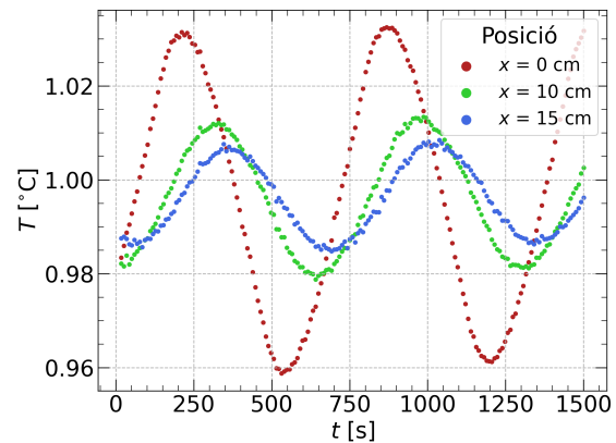
Figura 6: Gràfica de T en funció de t normalitzada de la barra gran. Temperatures mesurades a una distància de 0 cm (vermell), 10 cm (verd) i 15 cm (blau) del punt de referència.
