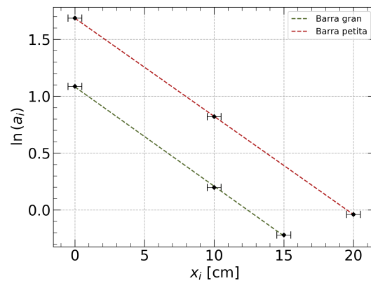
Figura 8: Regressió lineal del logaritme de les amplituds respecte a la posició. Coeficients de regressió obtinguts: r^2 = 0,999 tant per a la barra gran com per a la barra petita.
