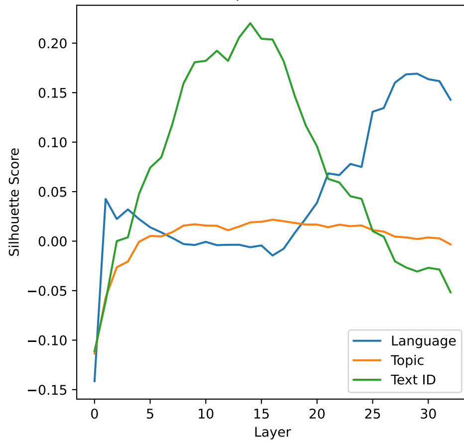
llama3-8b-cpt-sahabatai-v1-base
