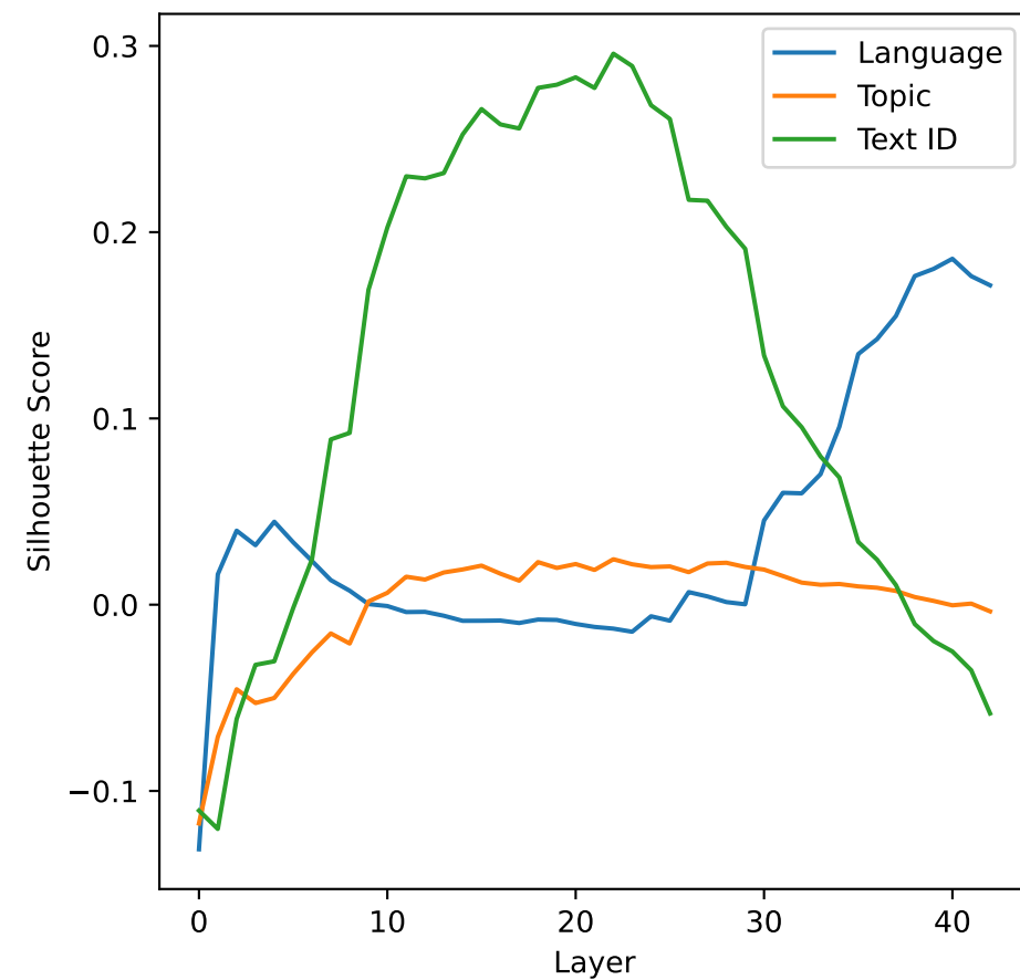
llama3-8b-cpt-sahabatai-v1-base
