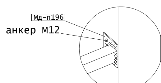
Узел 10
