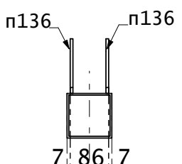
Разрез 509 - А
