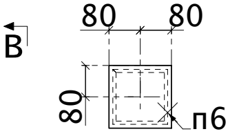
Вид 502-В
