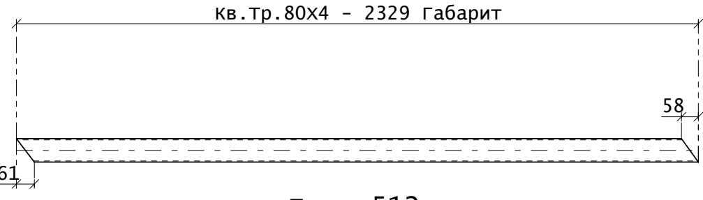
Поз. 512
