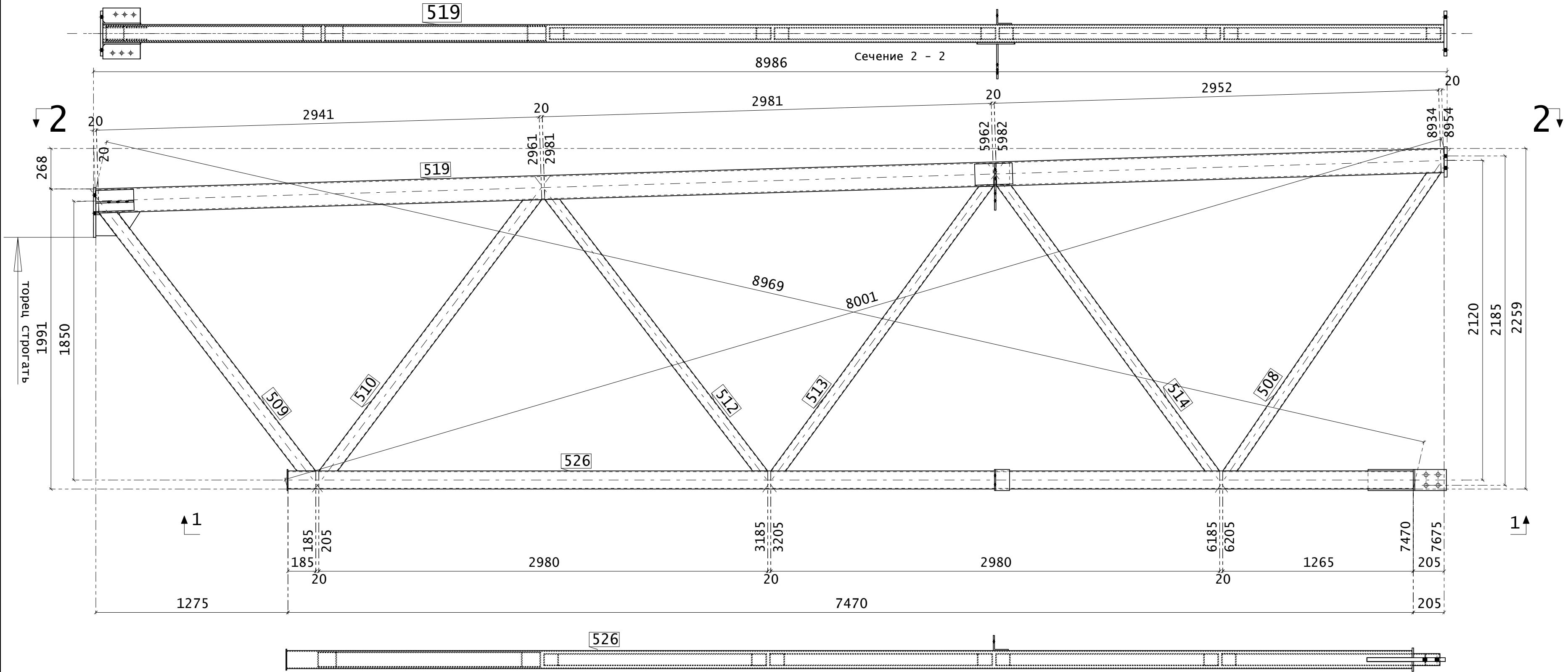
Сечение 1 - 1
