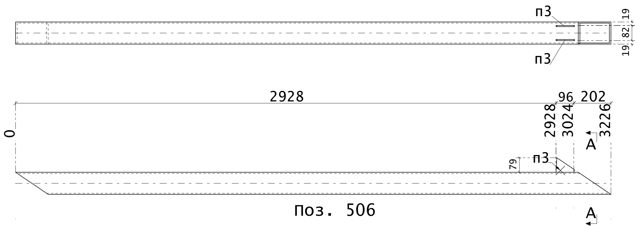
Разрез 506 - А
