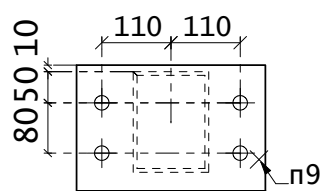
Вид 536-В
