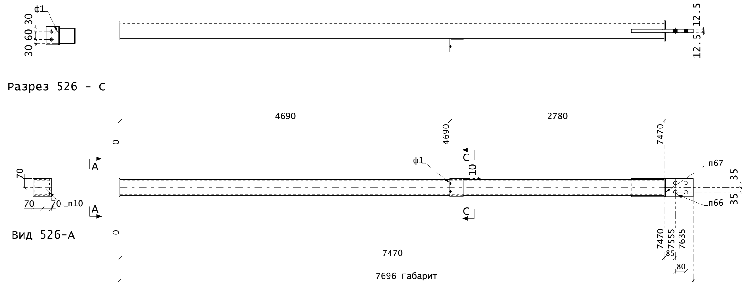
Поз. 526
