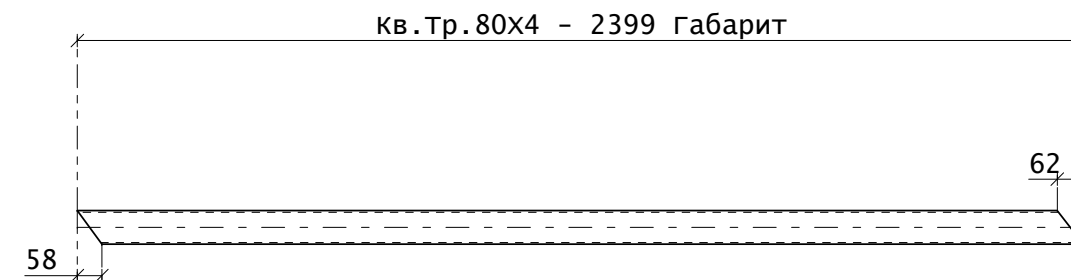
Поз. 513
