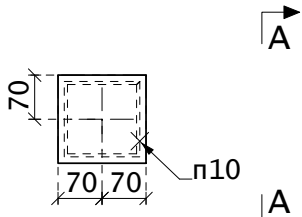
Вид 521-А
