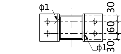
Разрез 521 - С
