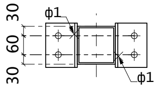
Разрез 521 - С
