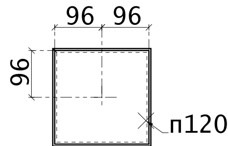
Вид В-В
