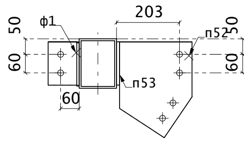
Разрез 545 - D
