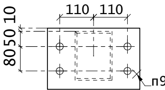
Вид 542-В
