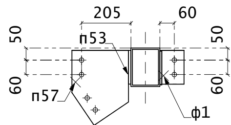
Разрез 546 – D
