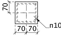
Вид 526-А
