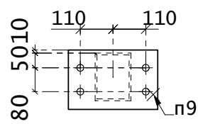
Вид 516-В
