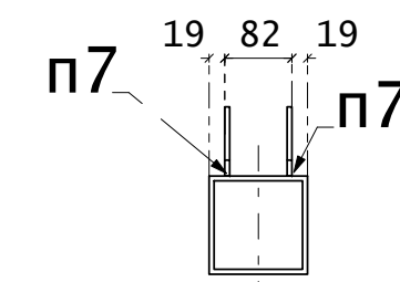
Разрез 501 - А
