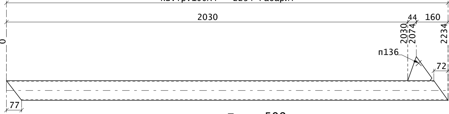
Поз. 509
