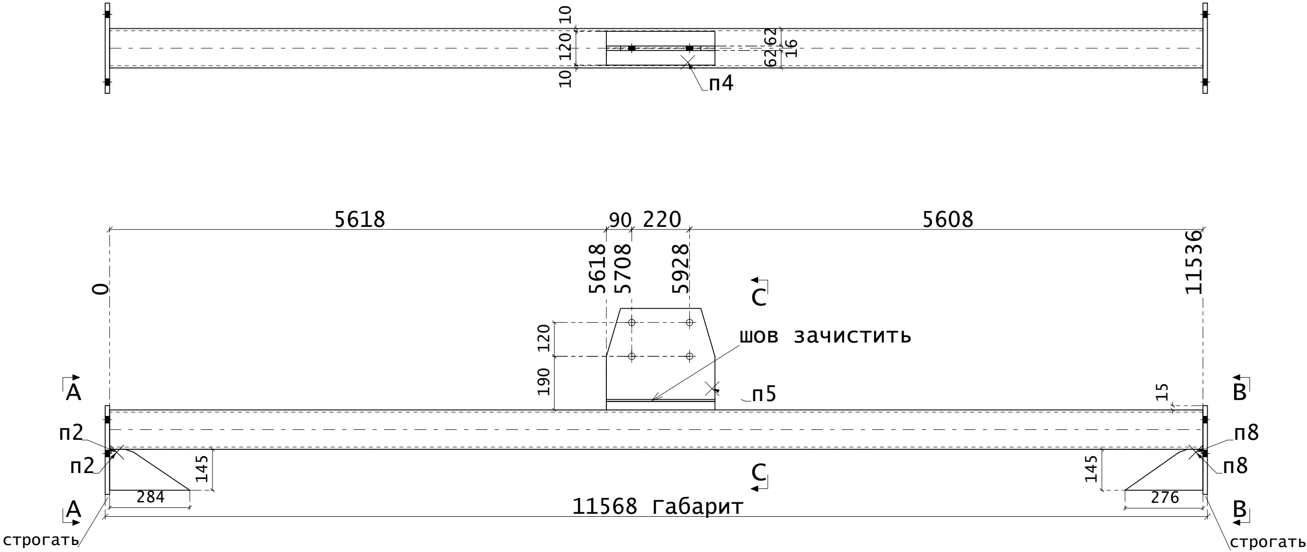
Поз. 503
