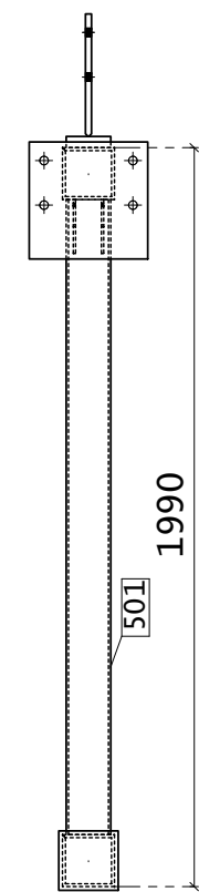
Сечение 1 - 1
