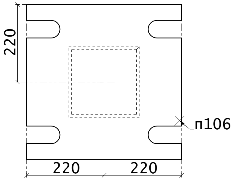
Вид А-А
