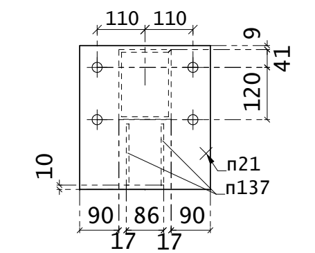
Вид 536-А
