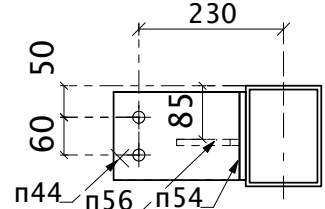
Разрез 542 - C
