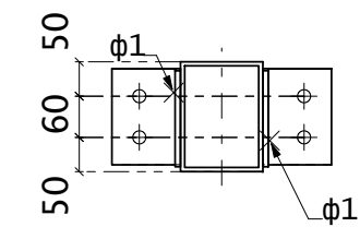
Разрез 536 - С
