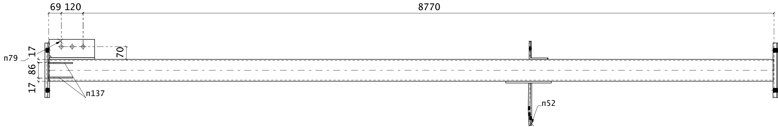
Поз. 545
