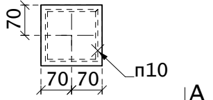
Вид 526-А
