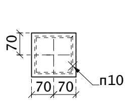
Вид 521-А
