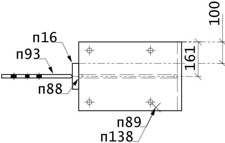
Разрез В - В
