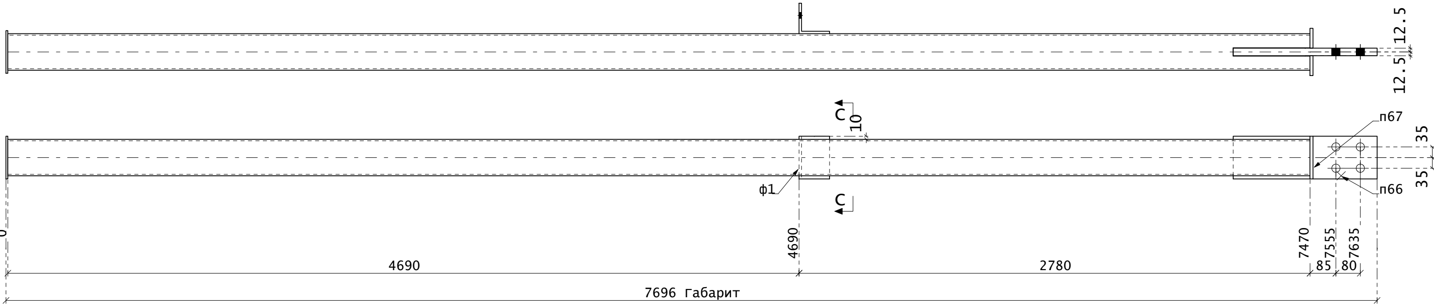
Поз. 527
