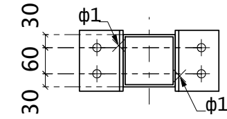
Разрез 521 - С
