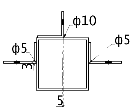
Разрез D - D
