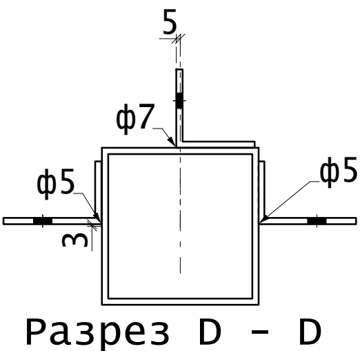
Разрез D - D
