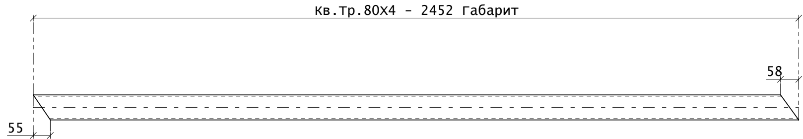
Поз. 508
