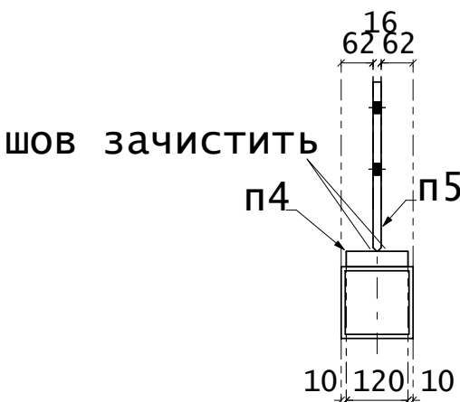
Разрез 503 - С
