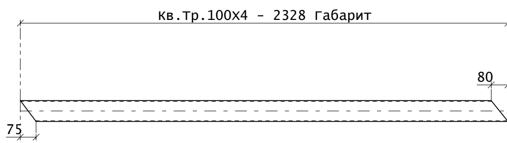
Поз. 510
