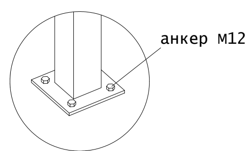
Узел 9
