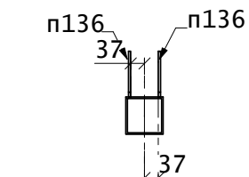
Разрез 509 - А
