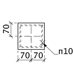
Вид 521-А
