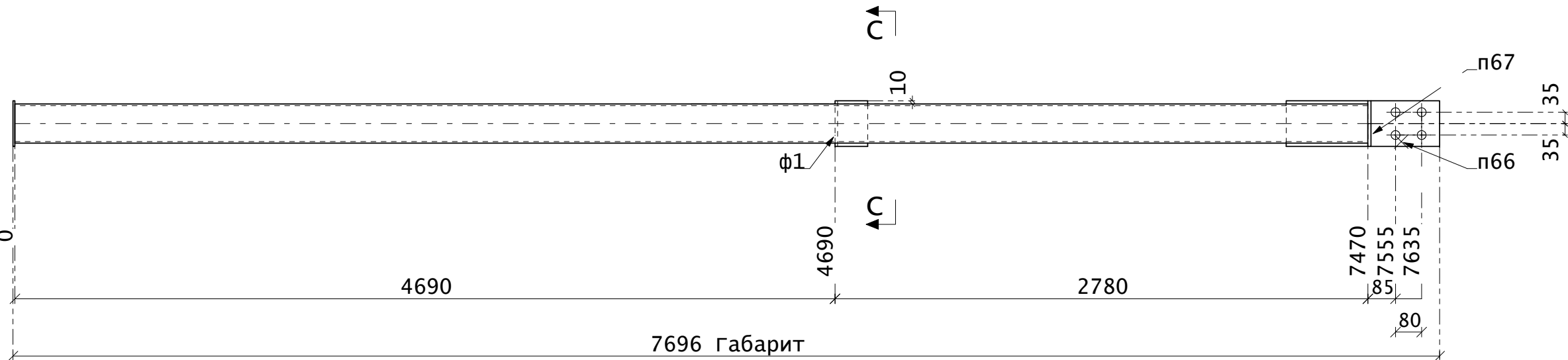
Поз. 527
