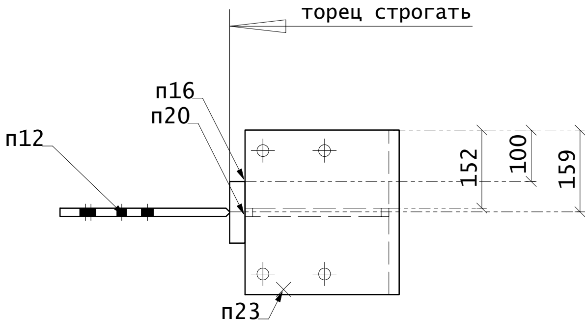
Вид А-А
