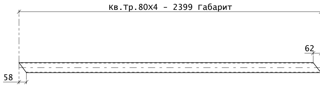
Поз. 513
