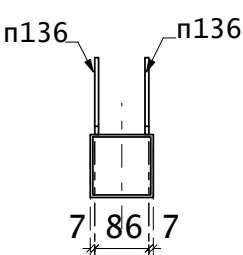
Разрез 509 - А
