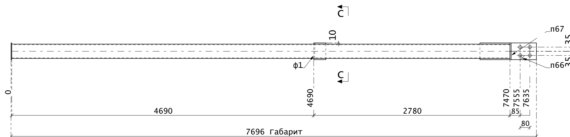
Поз. 527
