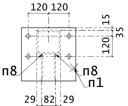
Вид 503-В
