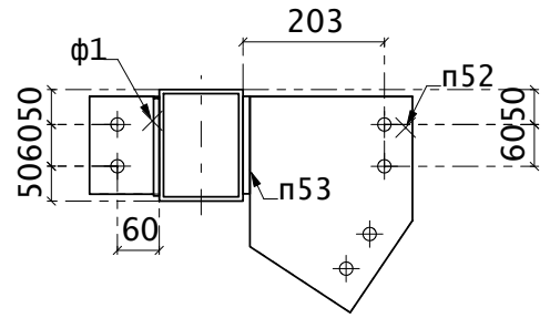
Разрез 545 - Д
