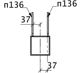
Разрез 509 - А
