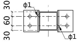
Разрез 521 - С
