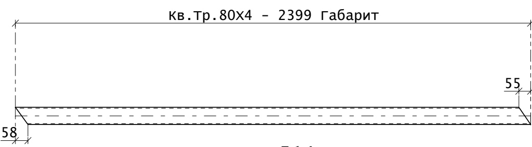
Поз. 514
