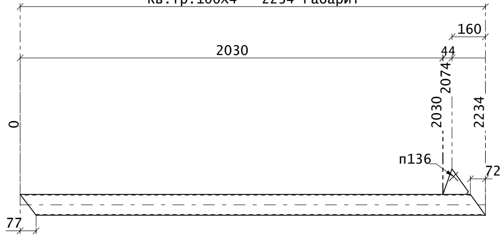
Поз. 509
