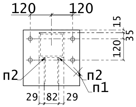
Вид 507-В
