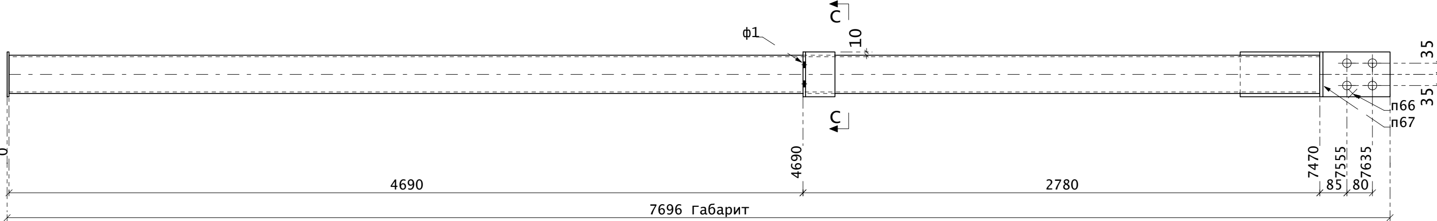
Поз. 521
