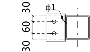
Разрез 526 - С
