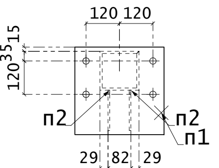
Вид 507-А
