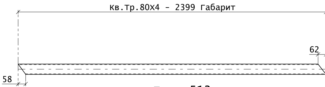
Поз. 513
