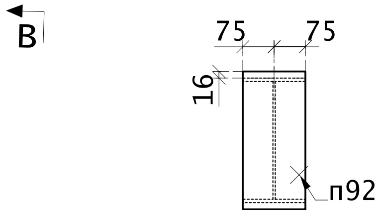
Вид 531-В
