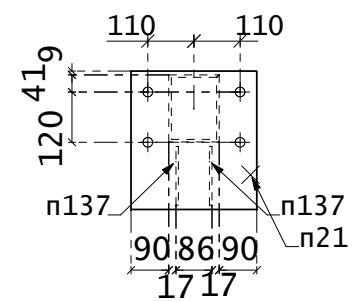
Вид 516-А
