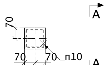
Вид 527-А
