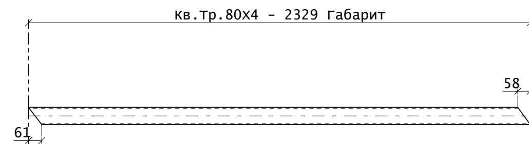
Поз. 512
