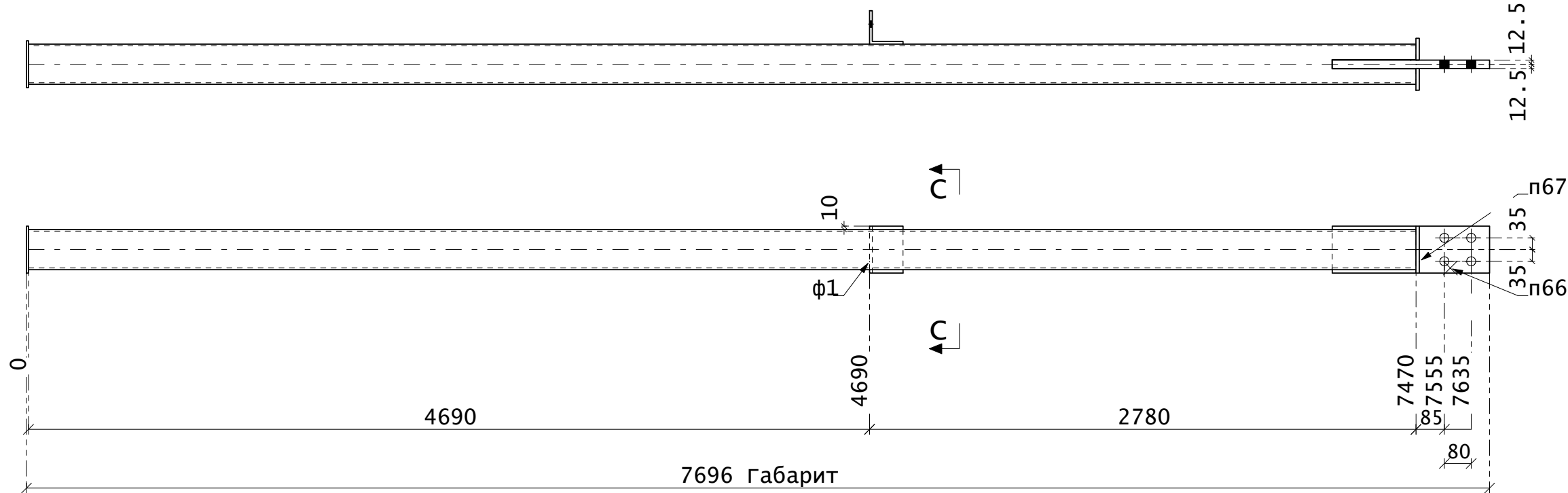
Поз. 527
