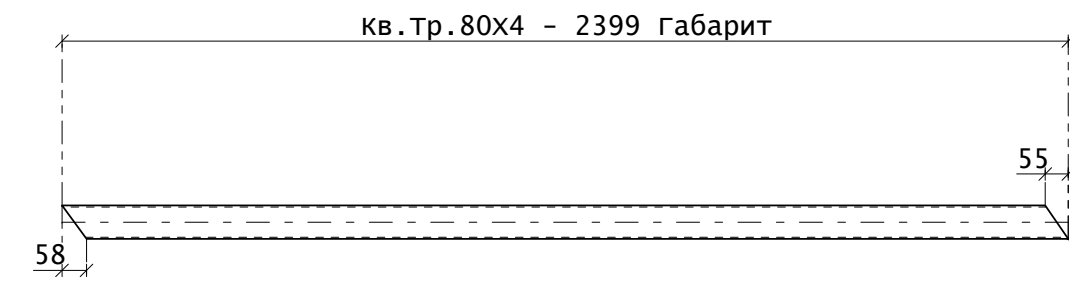
Поз. 514
