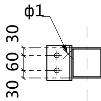
Разрез 526 - С
