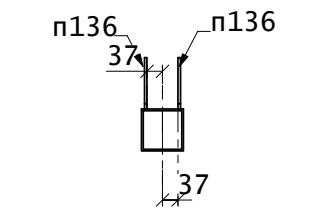
Разрез 509 - А
