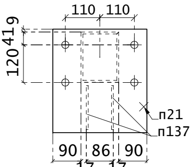
Вид 542-А
