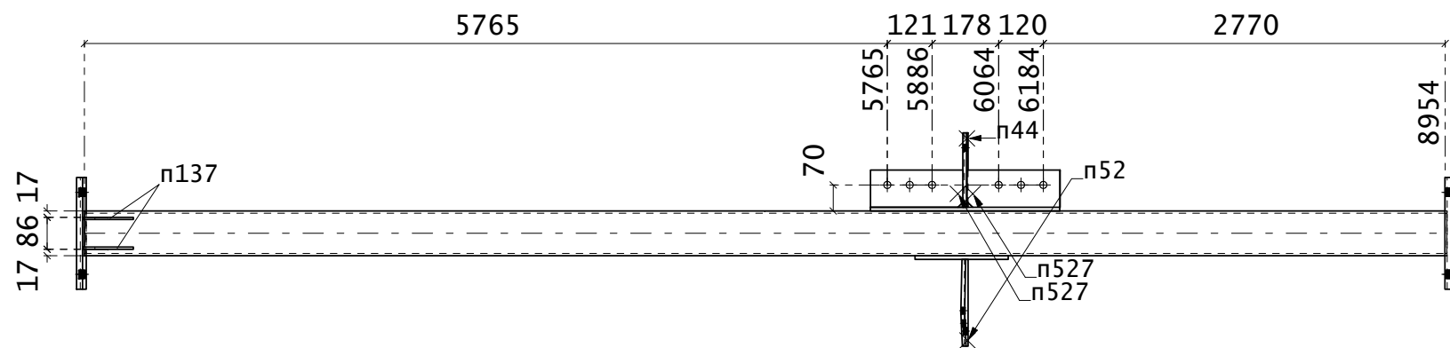
Поз. 516
