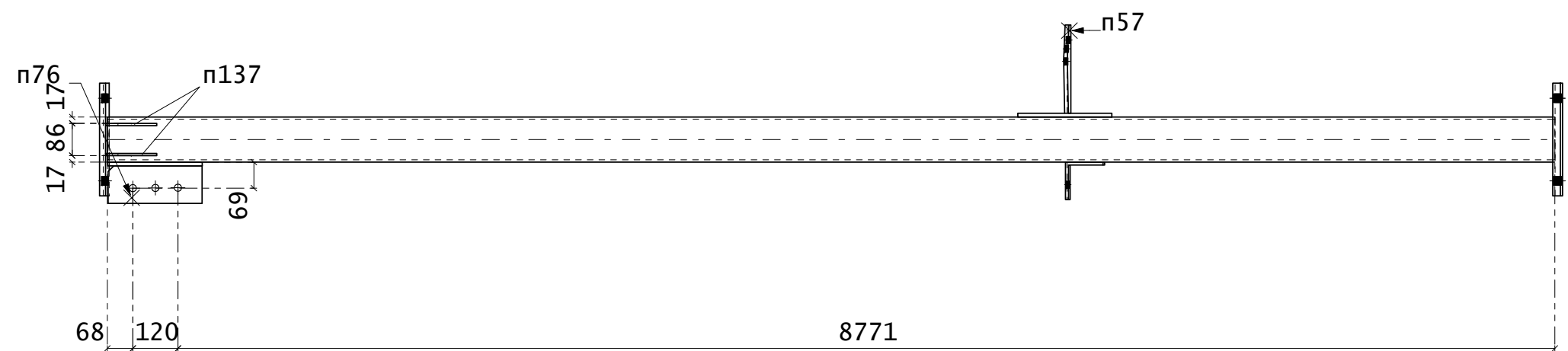
Поз. 546
