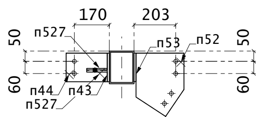
Разрез 516 - С
