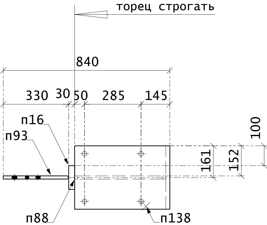
Вид А-А
