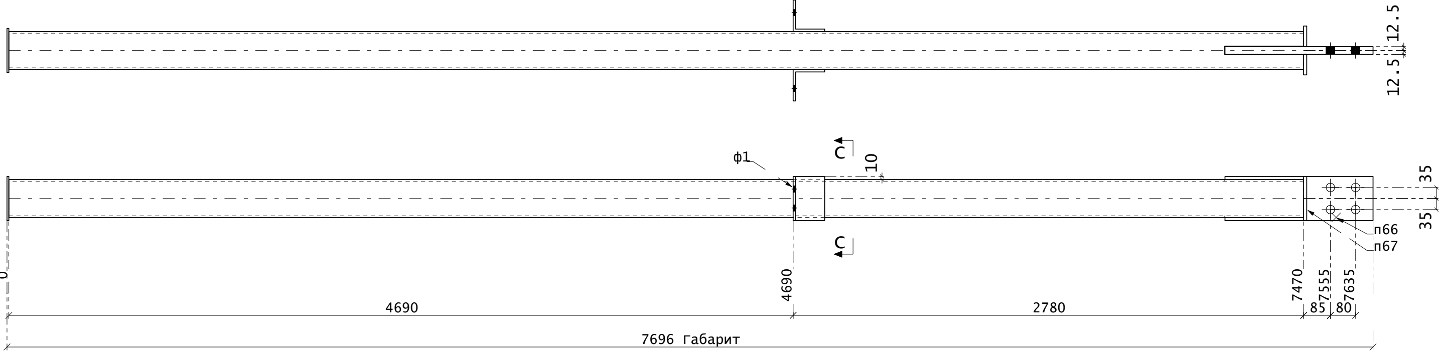
Поз. 521
