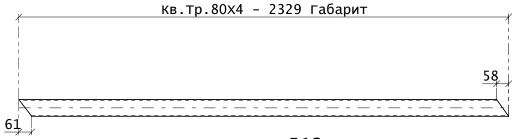
Поз. 512
