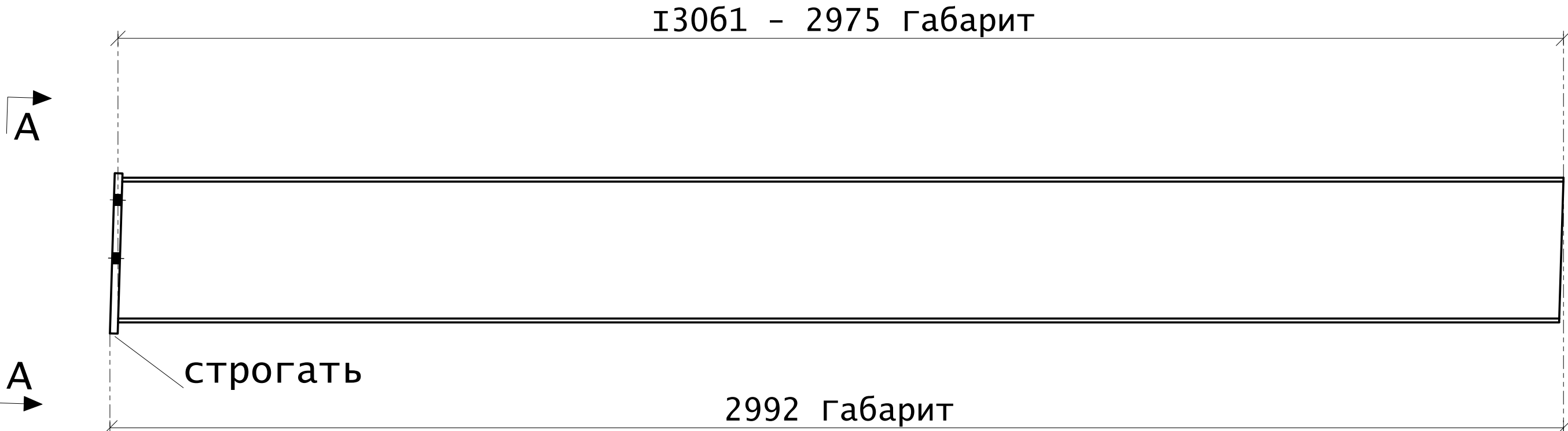
Поз. 525
