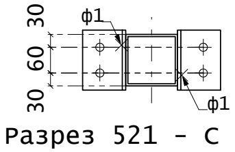
Разрез 521 - С
