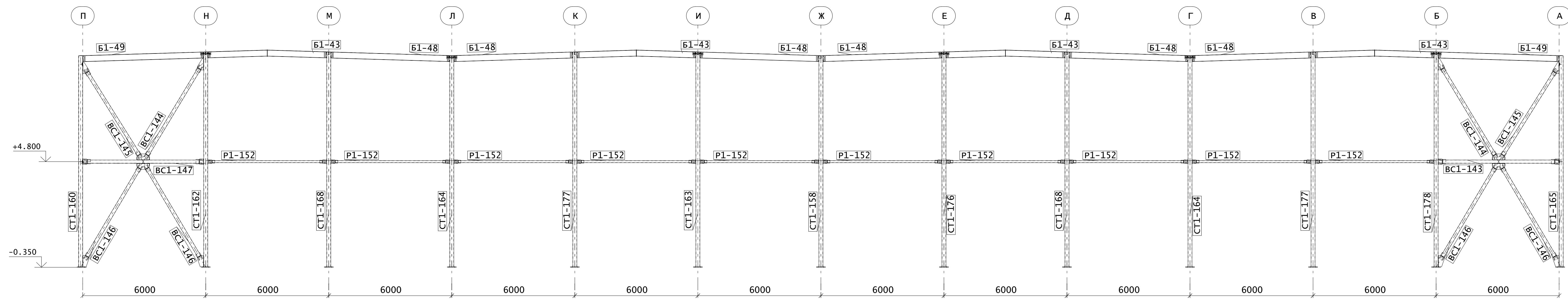
Разрез 5-5
