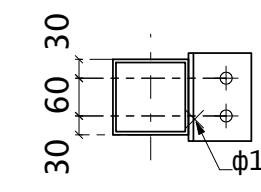
Разрез 527 - С
