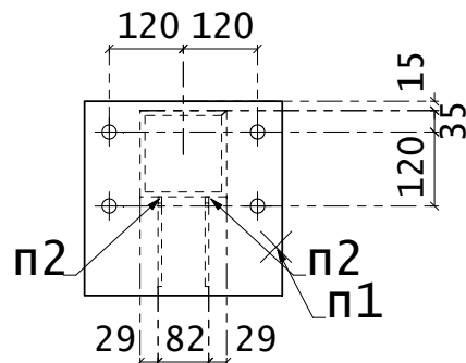
Вид 503-А
