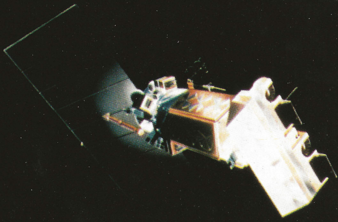
NOAA
