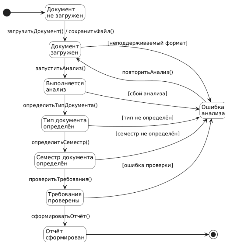
Рисунок 2.6 – Диаграмма состояний документа в системе
