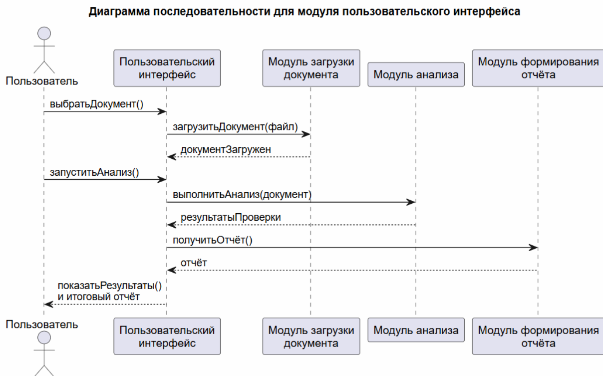
Рисунок 2.3 – Диаграмма последовательности взаимодействия пользователя с системой через интерфейс
