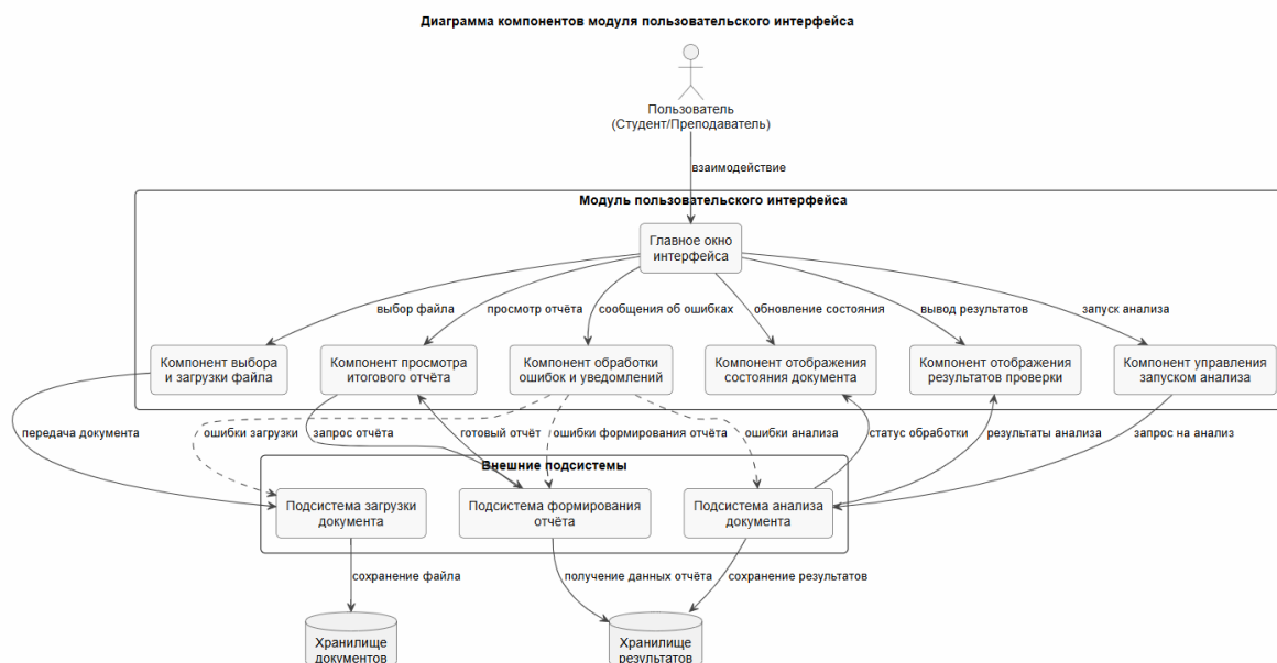
Рисунок 2.4 – Диаграмма компонентов модуля пользовательского интерфейса
