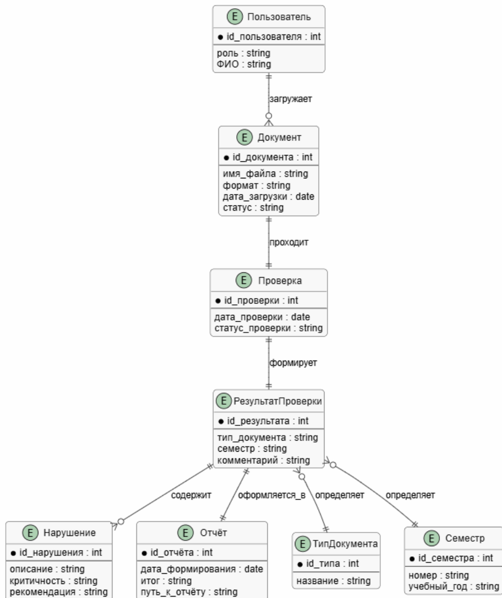
ER-диаграмма данных модуля пользовательского интерфейса
