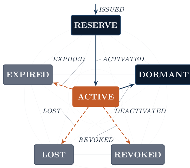
Рис. 3: Автомат жизненного цикла токена, не изменившийся с версии 1. ACTIVE есть единственное рабочее состояние. Токен входит через RESERVE , активируется и уходит через одно из трёх конечных состояний либо в DORMANT , когда дело принимает преемник. Законные переходы закреплены триггером trg_token_state_machine , и каждый переход автоматически записывает событие жизненного цикла.
