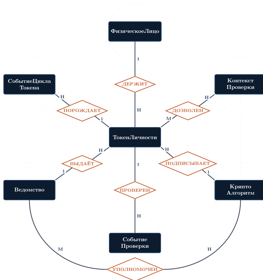
Рисунок 3 — Геометрия сущностей ядра, не изменившаяся с версии 1. Семь сущностей вокруг ТокенЛичности : человек, который его держит, ведомство, которое его выдаёт, алгоритм, который его подписывает, контексты, в которых он может проверяться, и два журнала событий, работающих только на добавление, которые он порождает. Связи «многие ко многим» разрешаются в соединительные таблицы ДопускКАлгоритму и РазрешениеТокена . Эта геометрия есть постоянная величина документа: раздел 4 рисует остальные тридцать восемь таблиц как кольца вокруг неё.
