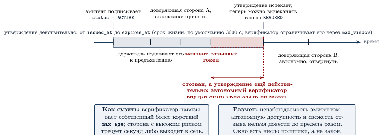
Рис. 7: Размен автономности, нарисованный как временная шкала. Эмитент подписывает утверждение о состоянии с окном; держатель подписывает его к предъявлению; доверяющая сторона, проверяющая автономно внутри окна, принимает. Если эмитент отзовёт удостоверение внутри окна, последнее утверждение ACTIVE останется действительным до истечения, и автономный верификатор об этом знать не может. Окно ограничено сроком жизни, выданным эмитентом (по умолчанию час), и величиной max_window , которую навязывает верификатор; доверяющая сторона с высоким риском требует секунд либо выходит в сеть.
