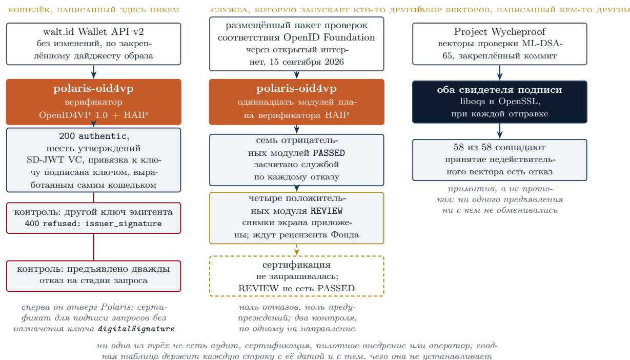
Рис. 6: Три вещи за пределами репозитория, которые его задействовали, и два контроля, без которых первая из них ничего бы не значила. Кошелек, написанный здесь никем, предъявил удостоверение и был принят; тот же кошелек, когда верификатор доверял другому ключу эмитента, получил отказ; и повторное предъявление против уже отвеченного запроса получило отказ. Размещённый пакет Фонда сам засчитал семь отказов и оставил четыре принятия на человека-рецензента. Опубликованный набор векторов сходится с обоими свидетелями подписи на примитиве. Ни одна из трёх не есть аудит, сертификация или пилотное внедрение.
