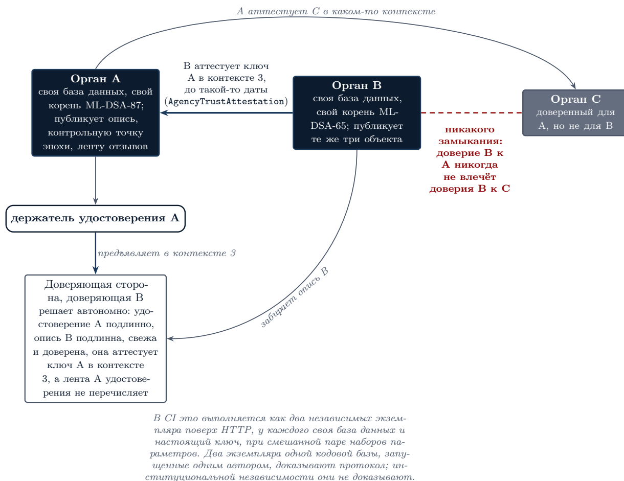
Рис. 9: Два органа и одна направленная аттестация. В аттестует ключ А в одном контексте; доверяющая сторона, доверяющая В, принимает удостоверение А в этом контексте, автономно, из описи В и ленты отзывов А. А доверяет также С, и В это не даёт ничего: доверие никогда не есть замыкание. В СИ это выполняется как два независимых экземпляра поверх HTTP при смешанной паре наборов параметров.
