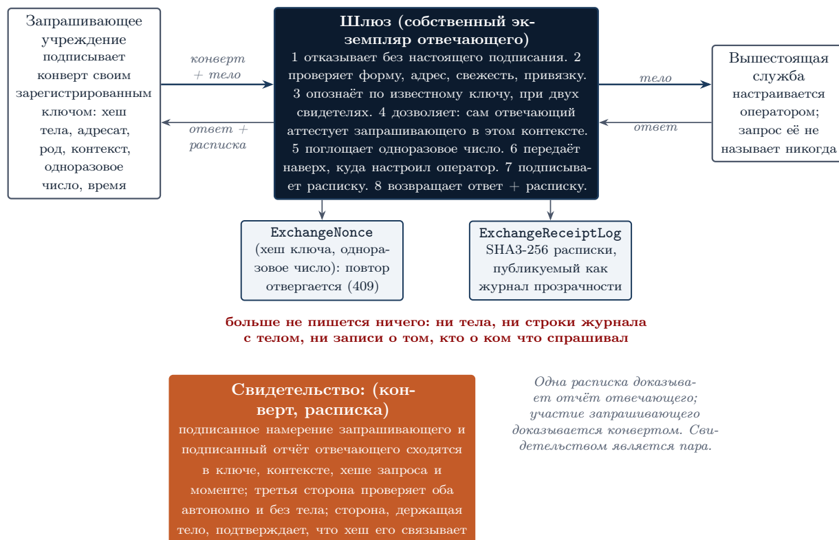
Рис. 11: Ведомственный обмен через шлюз. Запрашивающий подписывает конверт своим зарегистрированным ключом; собственный экземпляр отвечающего опознаёт его по ключу, который уже знает, позволяет его через собственную аттестацию в контексте конверта ещё до того, как что-либо покинет процесс, поглощает одноразовое число в регистре повторов, работающем только на добавление, передаёт тело лишь той вышестоящей службе, которую настроил оператор, и возвращает ответ с подписанной распиской. Не пишется ничего, кроме хеша расписки и поглощённого одноразового числа. Свидетельством обмена служит пара из конверта и расписки, проверяемая автономно третьей стороной и без всякого тела.
