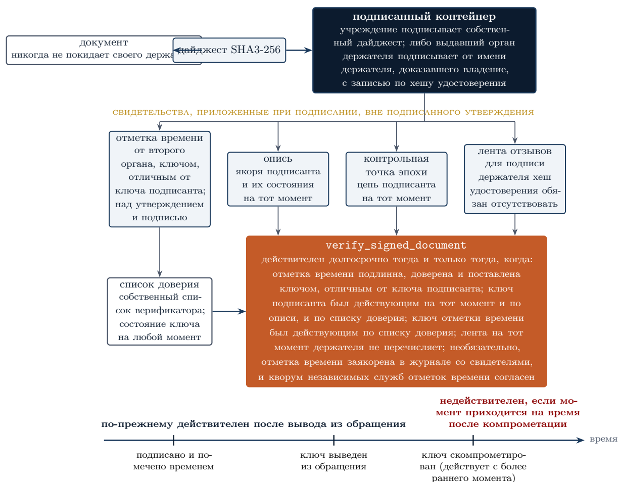
Рис. 12: Подписанный документ и его долгосрочные свидетельства. Документ никогда не покидает своего держателя; его дайджест подписывает учреждение либо выдающий орган держателя от имени держателя после доказательства владения, с записью по хешу удостоверения. Свидетельства, закреплённые в момент подписания, а именно отметка времени от отличного ключа, опись подписанта, его контрольная точка и лента, вместе с собственным списком доверия верификатора позволяют верификатору решить вопрос о действительности на тот момент спустя долгое время после вывода подписывающего ключа из обращения. Подпись, момент которой приходится на время после компрометации, отвергается, даже если вложенная в неё опись говорит, что ключ был действующим.
