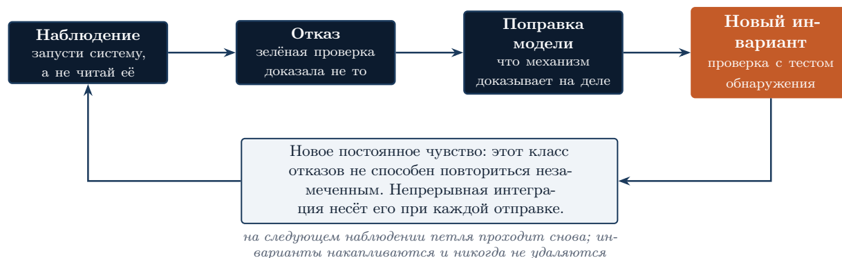
Рисунок 14 — Петля, которой ошибка становится постоянным чувством. Наблюдение есть запуск системы, а не её чтение; отказ есть зелёная проверка, доказавшая не то; поправка есть новая формулировка того, что механизм доказывает; инвариант есть проверка с тестом обнаружения; и с этого момента непрерывная интеграция несёт его при каждой отправке.
