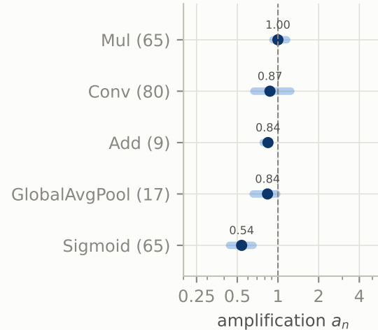
EfficientNet-B0
