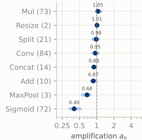
YOLOv10-S
