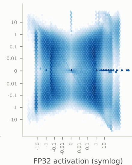
YOLOv10-S
