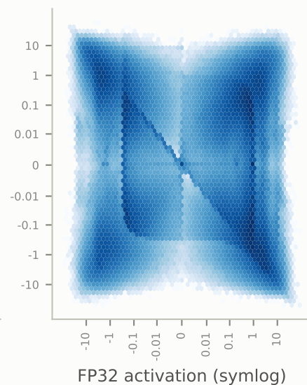
EfficientNet-B0
