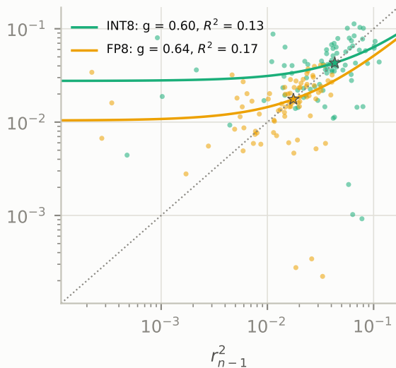
YOLOv10-S
